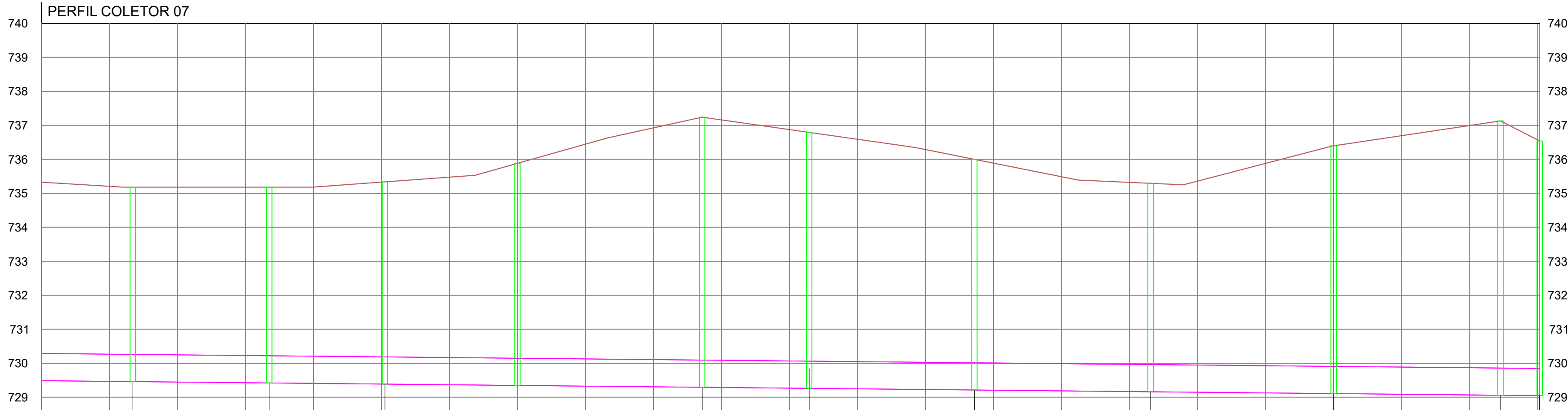
PERFIL COLETOR 07
