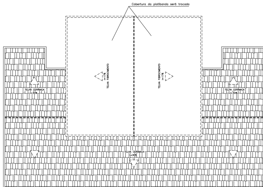
PLANTA DA COBERTURA Escala.....1 : 100
