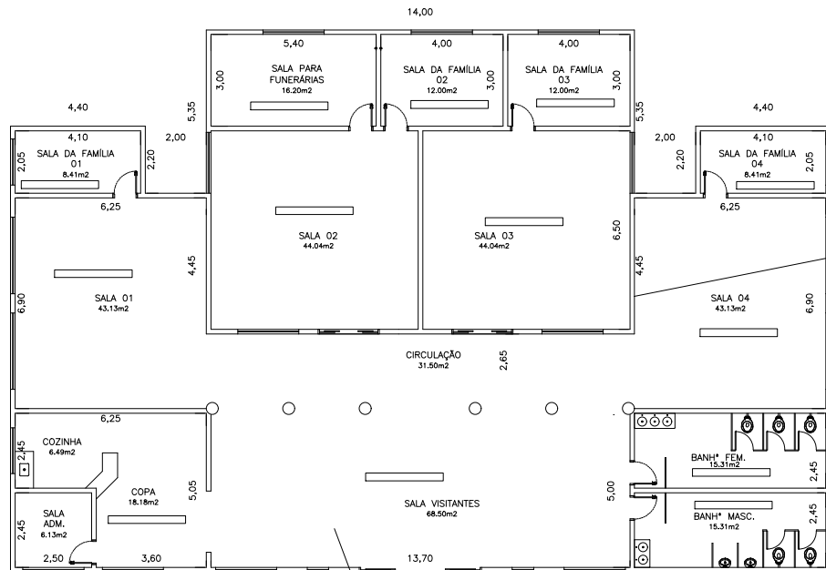
PLANTA Escala.....1 : 100
