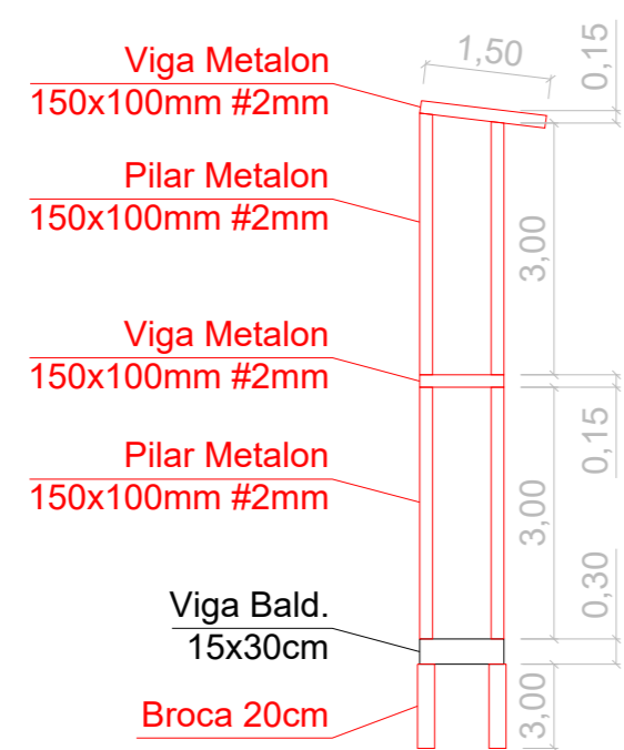
CORTE ESTRUTURA PARA ELEVADOR ESC. 1:100
