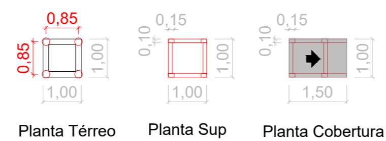
PLANTAS ESTRUTURA PARA ELEVADOR ESC. 1:100
