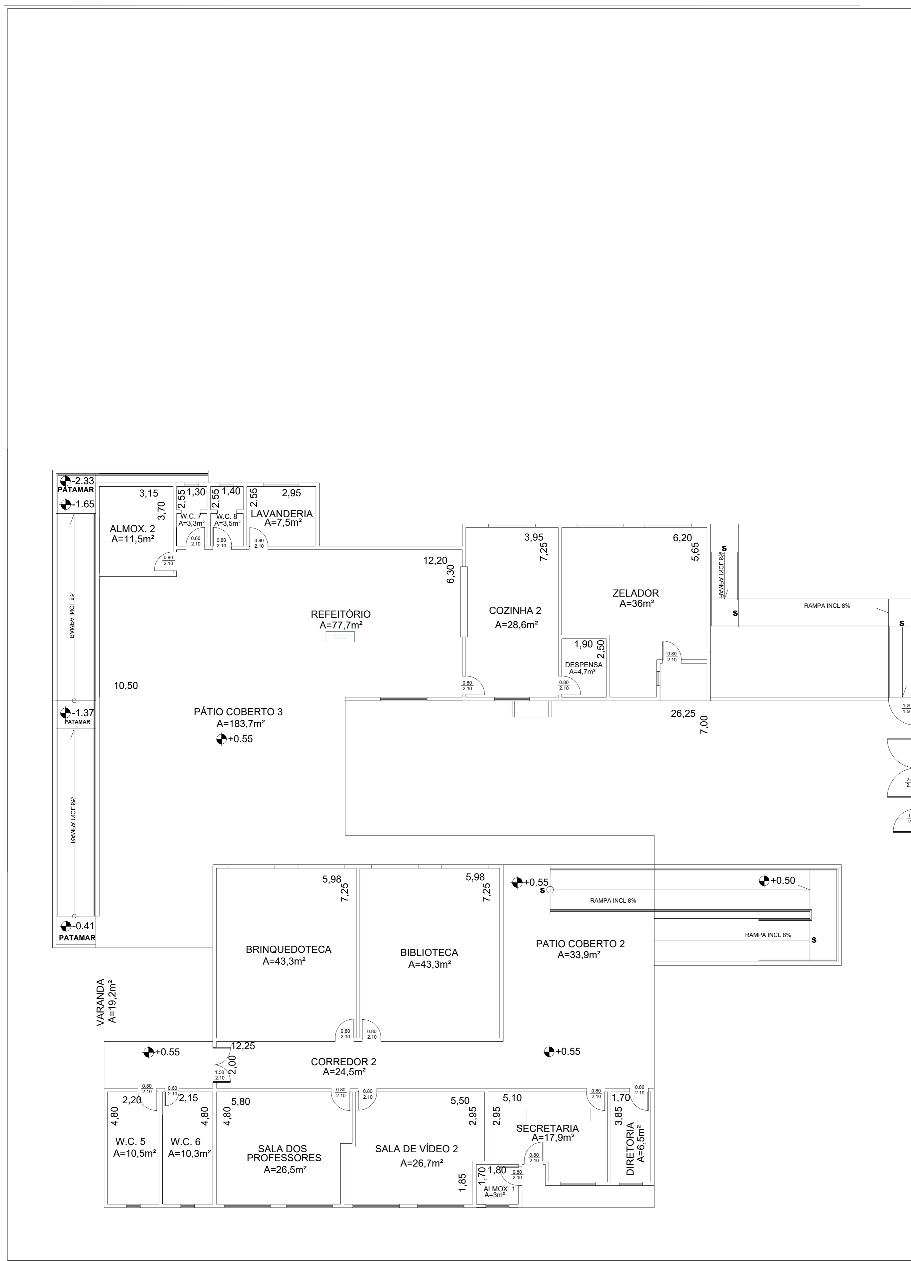
PLANTA TÉRREO ESC. 1:100
