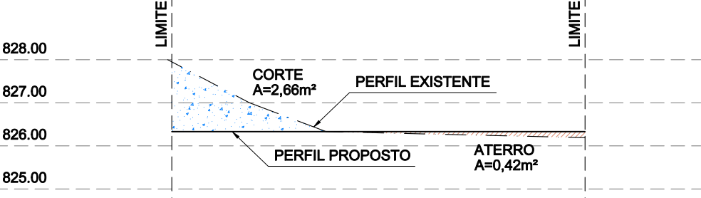
PERFIL H'H'
