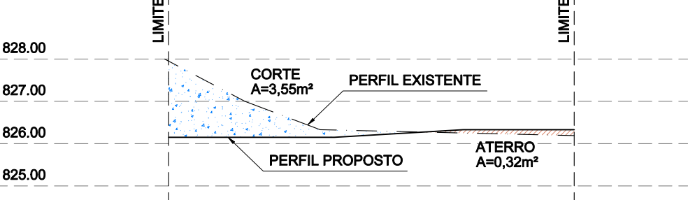
PERFIL HH
