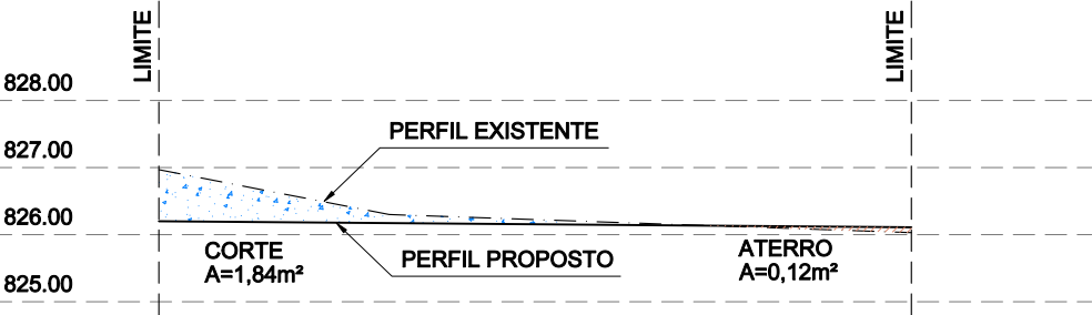
PERFIL G'G'
