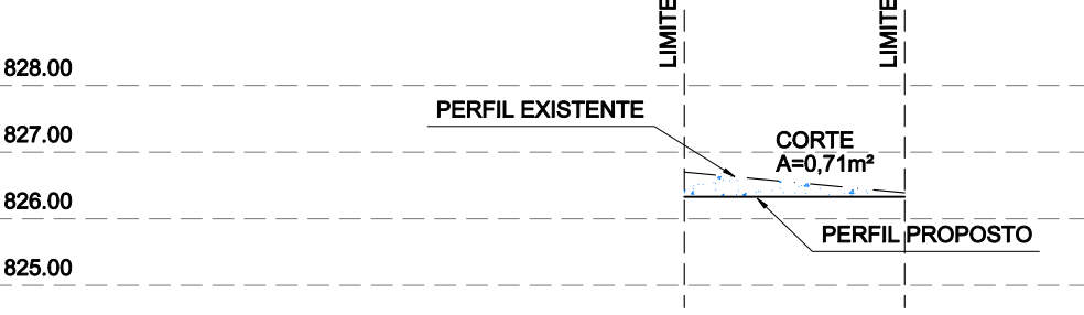
PERFIL JJ
