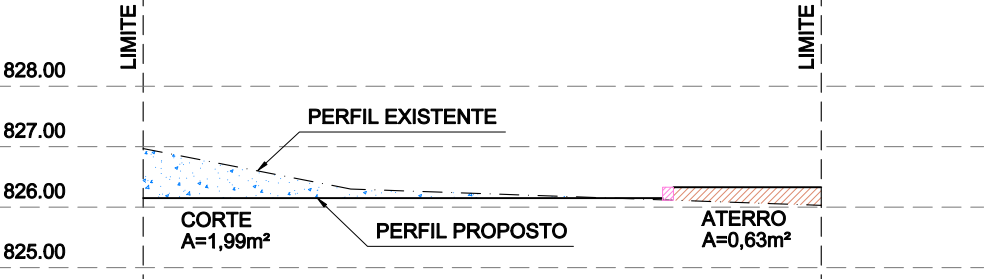
PERFIL GG
