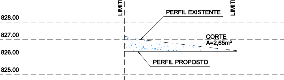
PERFIL II
