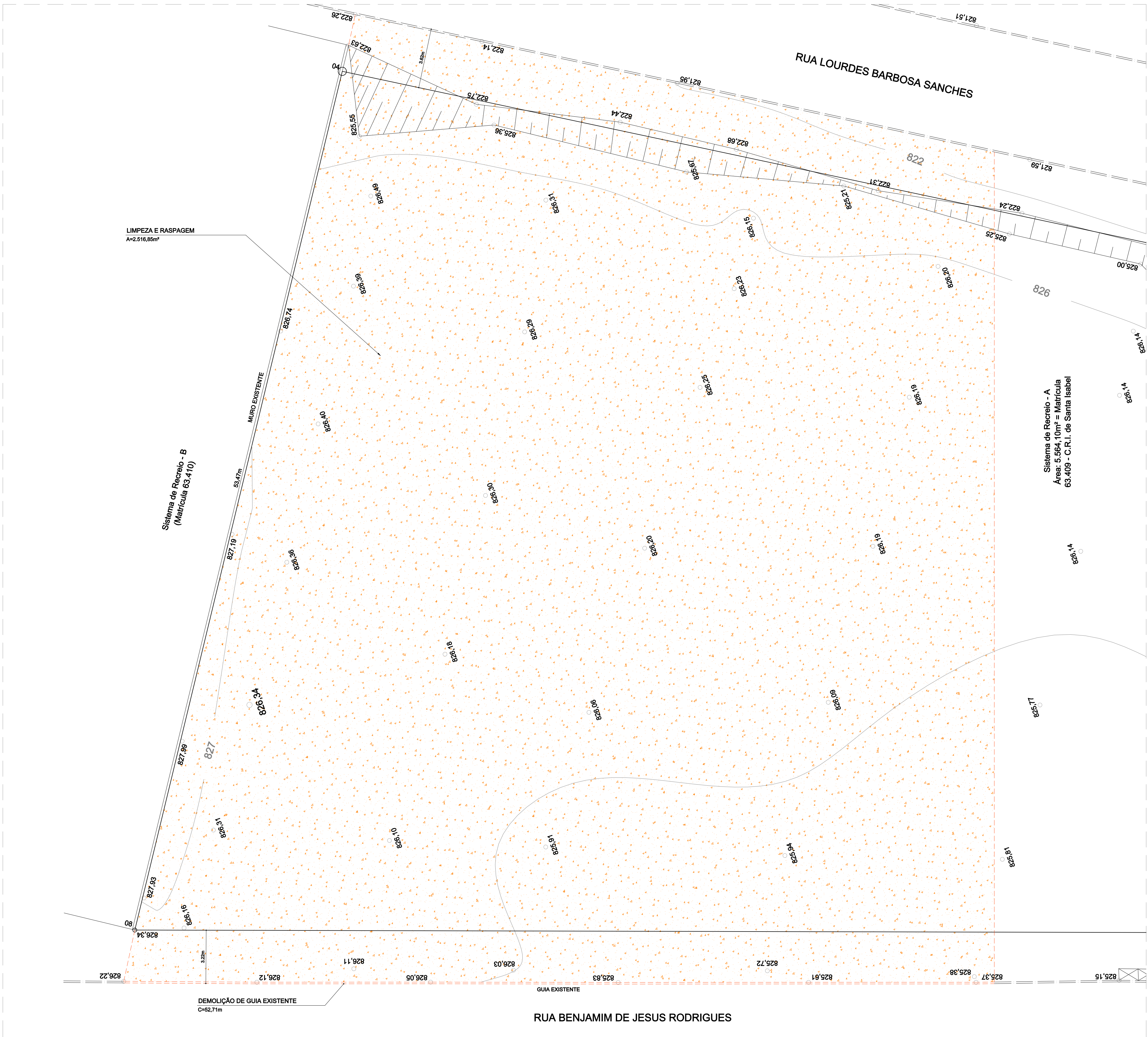
PLANTA DE DEMOLIÇÕES E RETIRADAS ESC. 1:125
