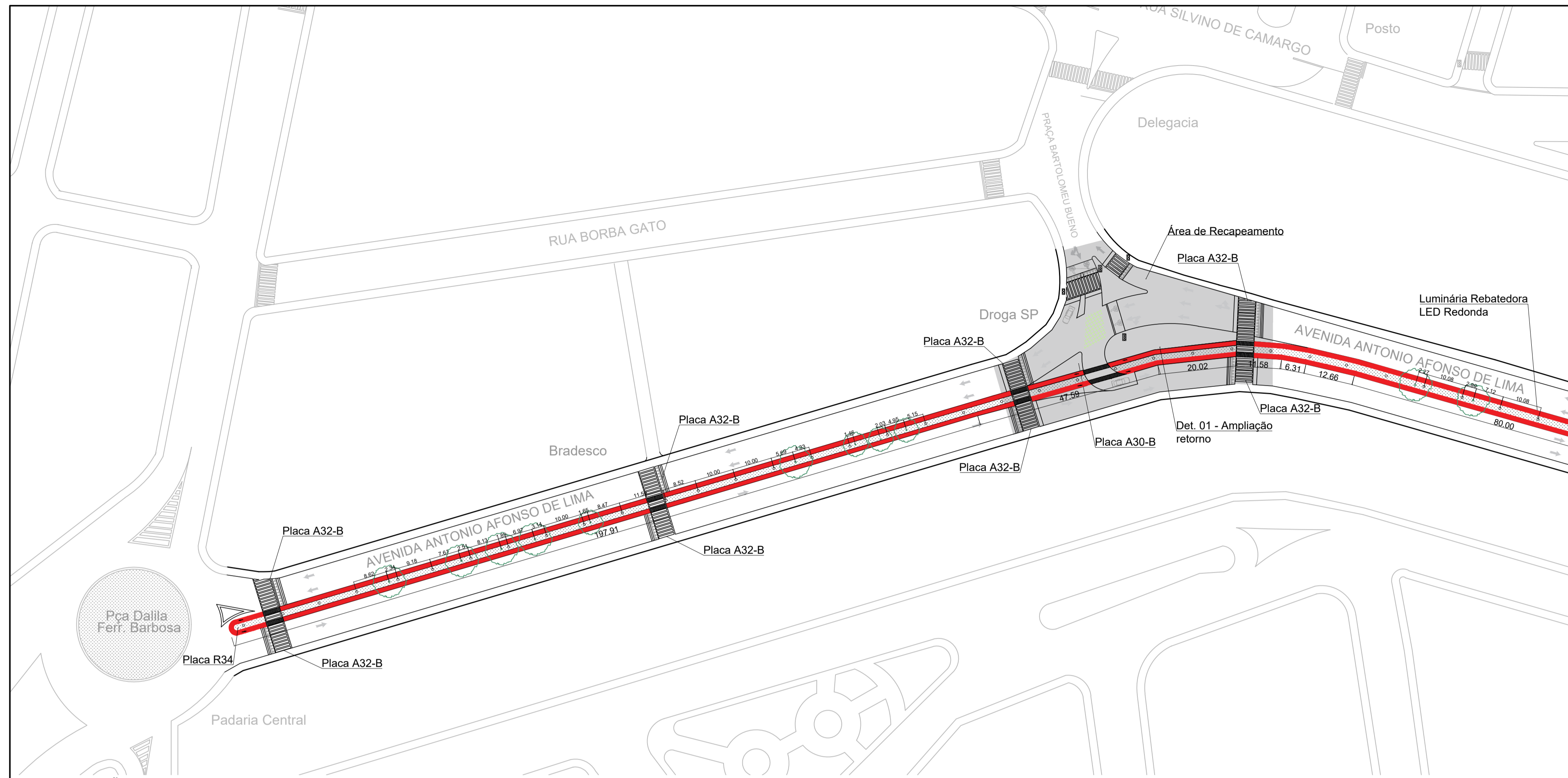
IMPLANTAÇÃO TRECHO 01 1:750
