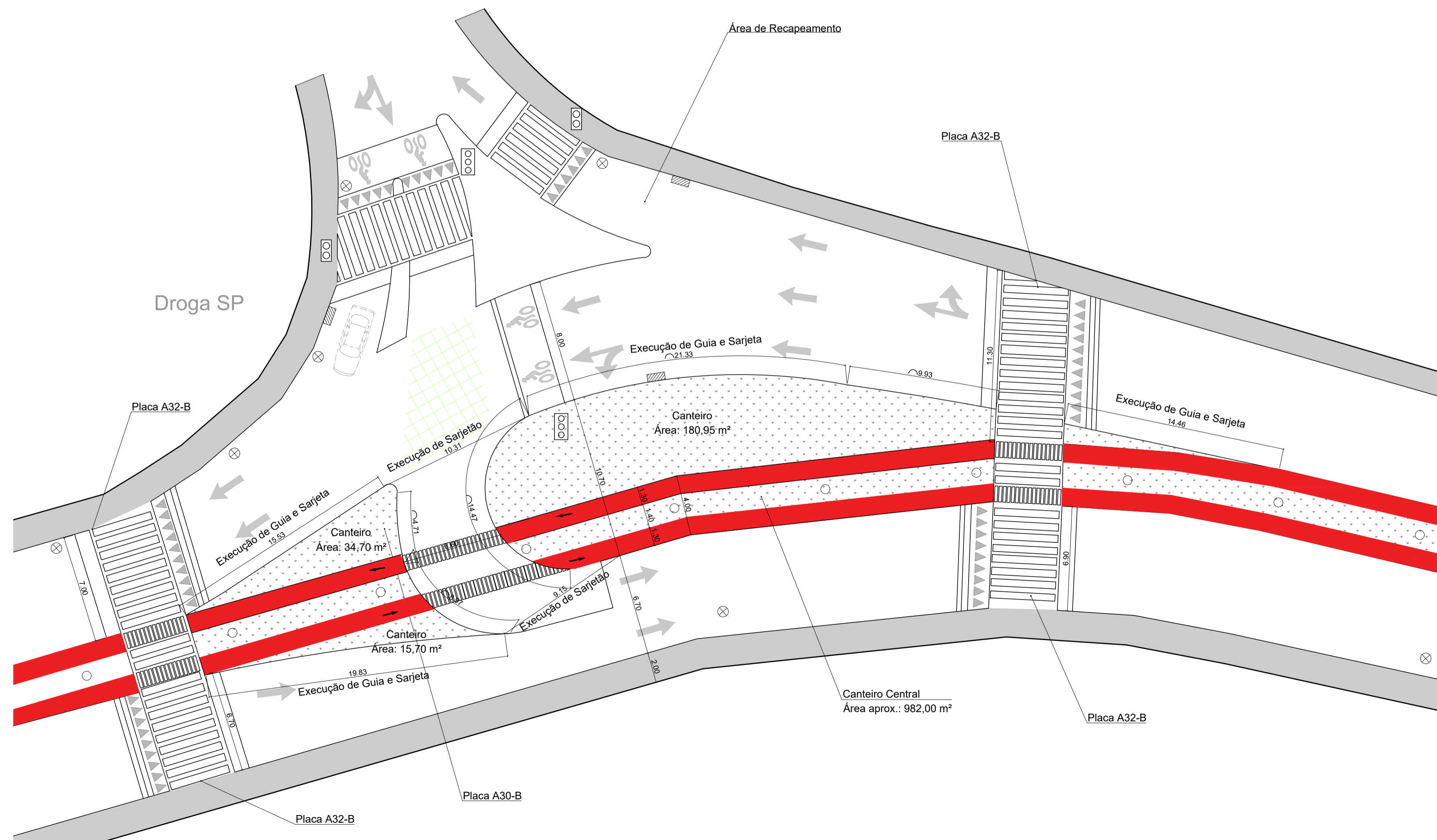
DET. 01 - AMPLIAÇÃO RETORNO 1:200
