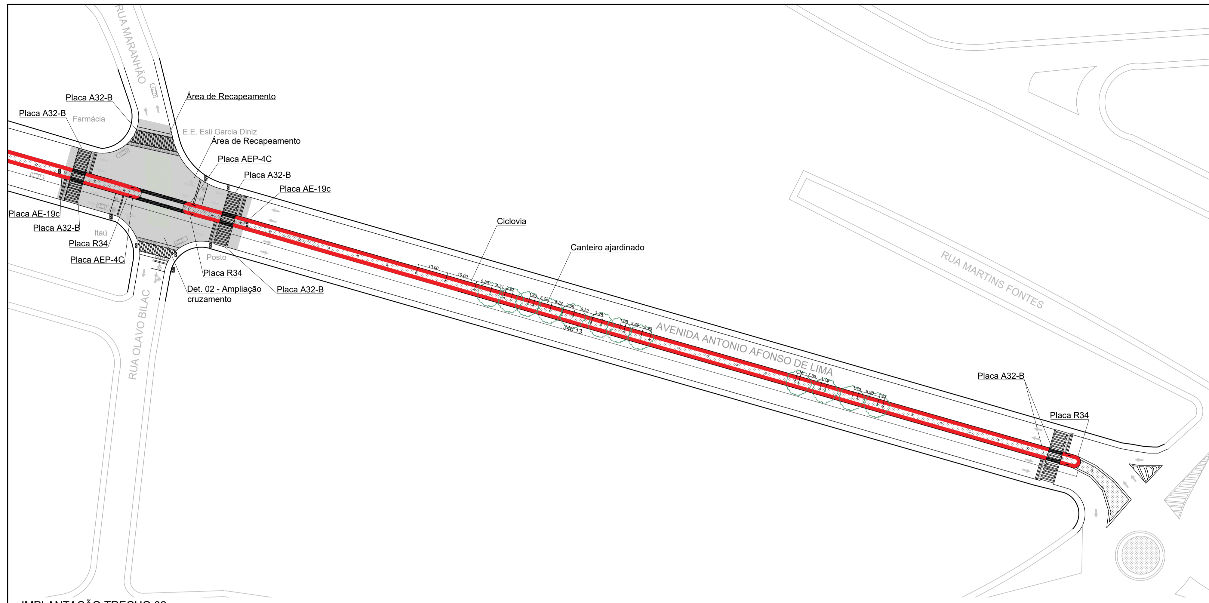
IMPLANTAÇÃO TRECHO 02 1:750
