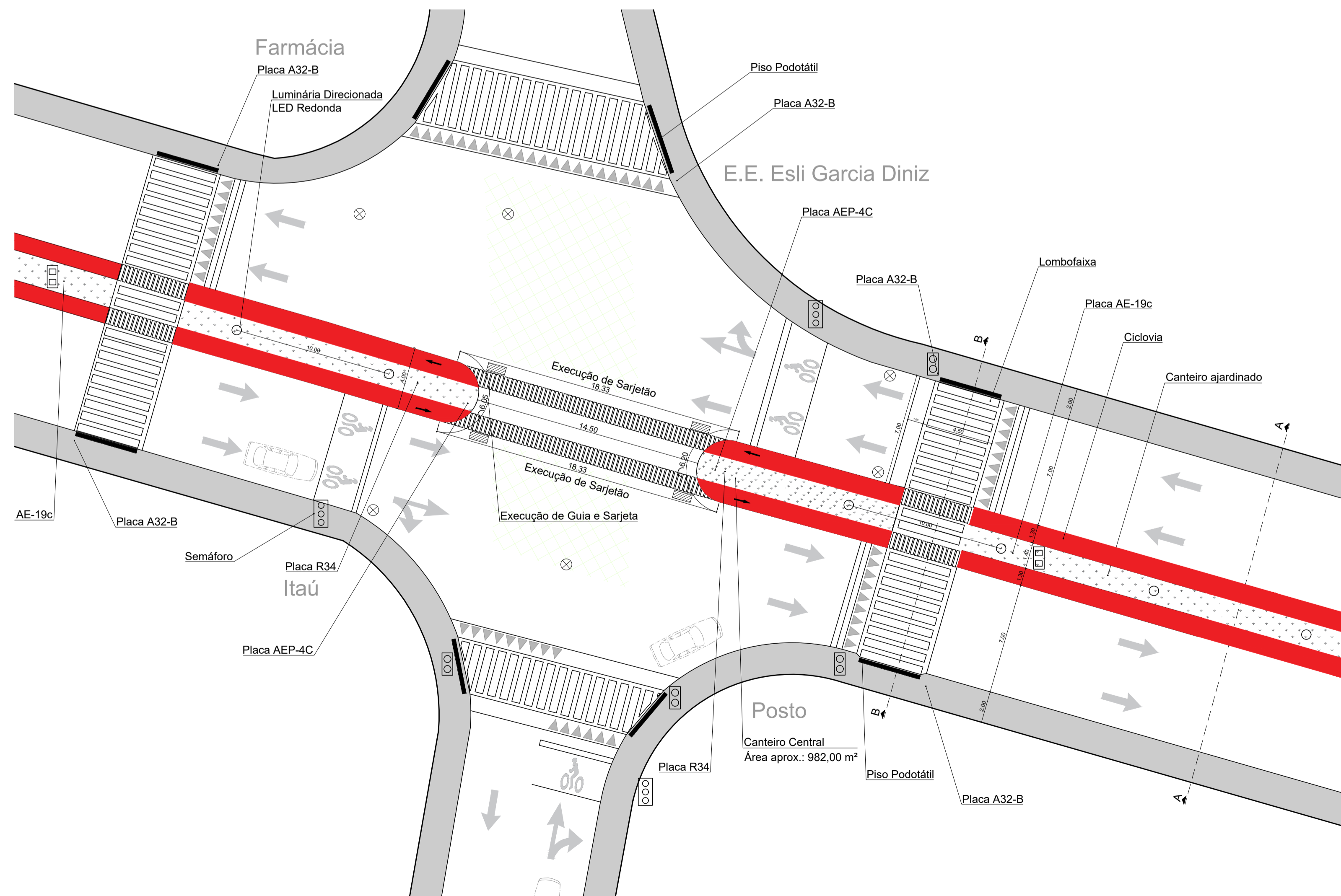
DET. 02 - AMPLIAÇÃO CRUZAMENTO 1:200
