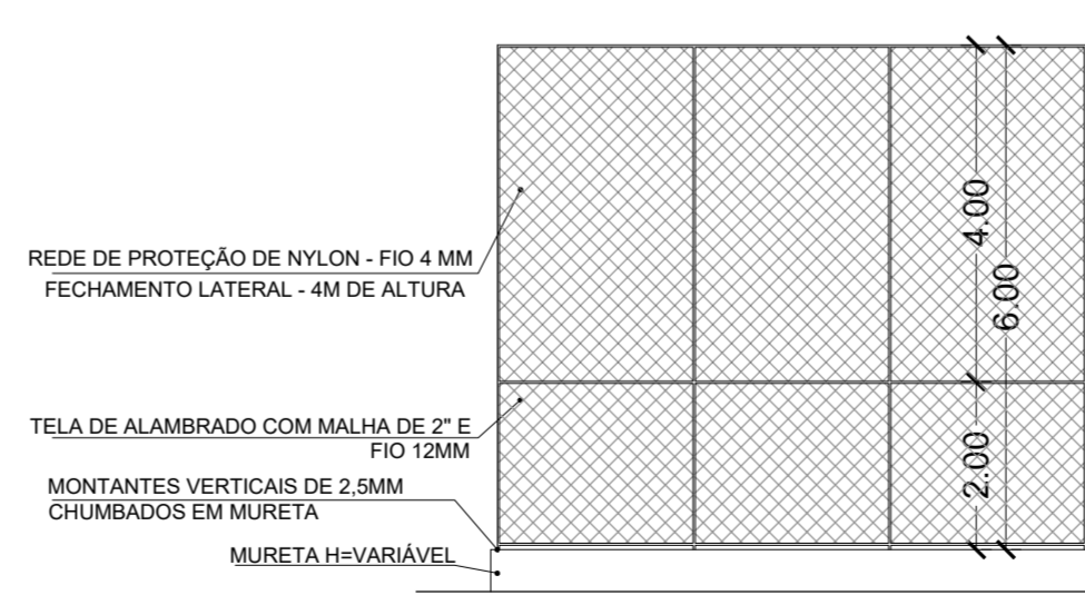
DET. 01 - VISTA FECHAMENTO LATERAL ESC. 1:100
