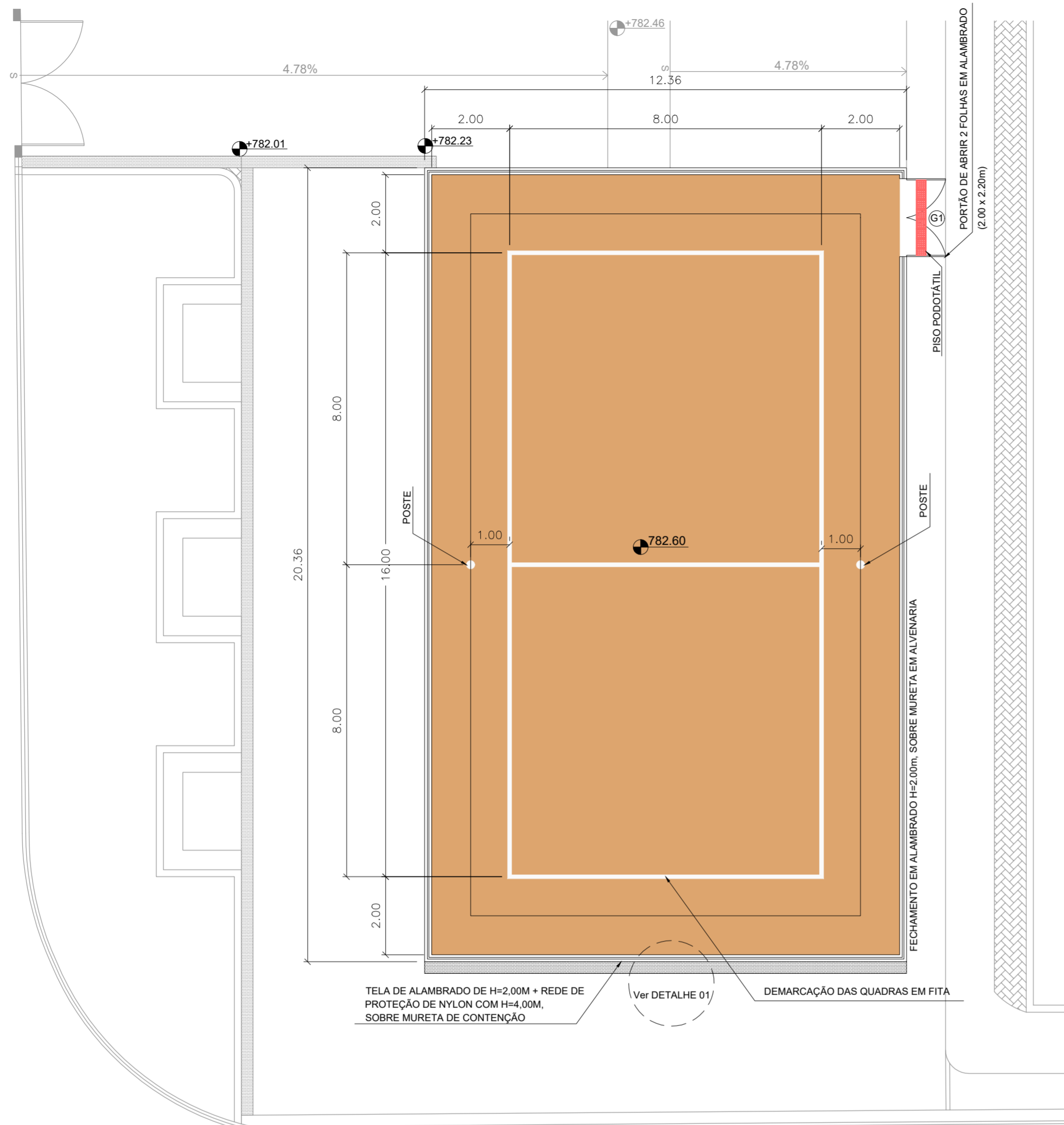
PLANTA TÉCNICA ESC. 1:100
