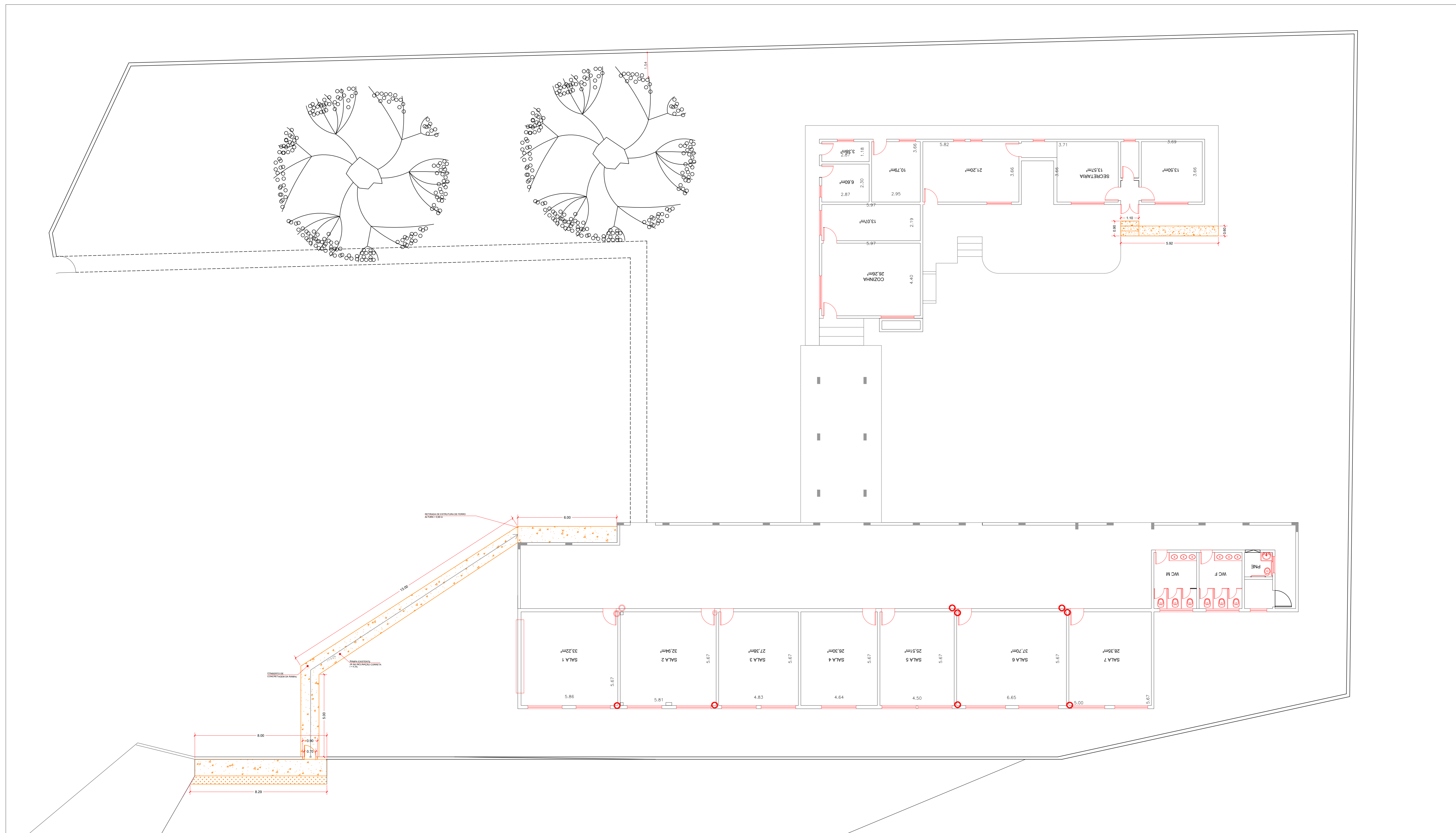
PLANTA CADASTRO/ DEMOLIÇÃO Escala 1:100
