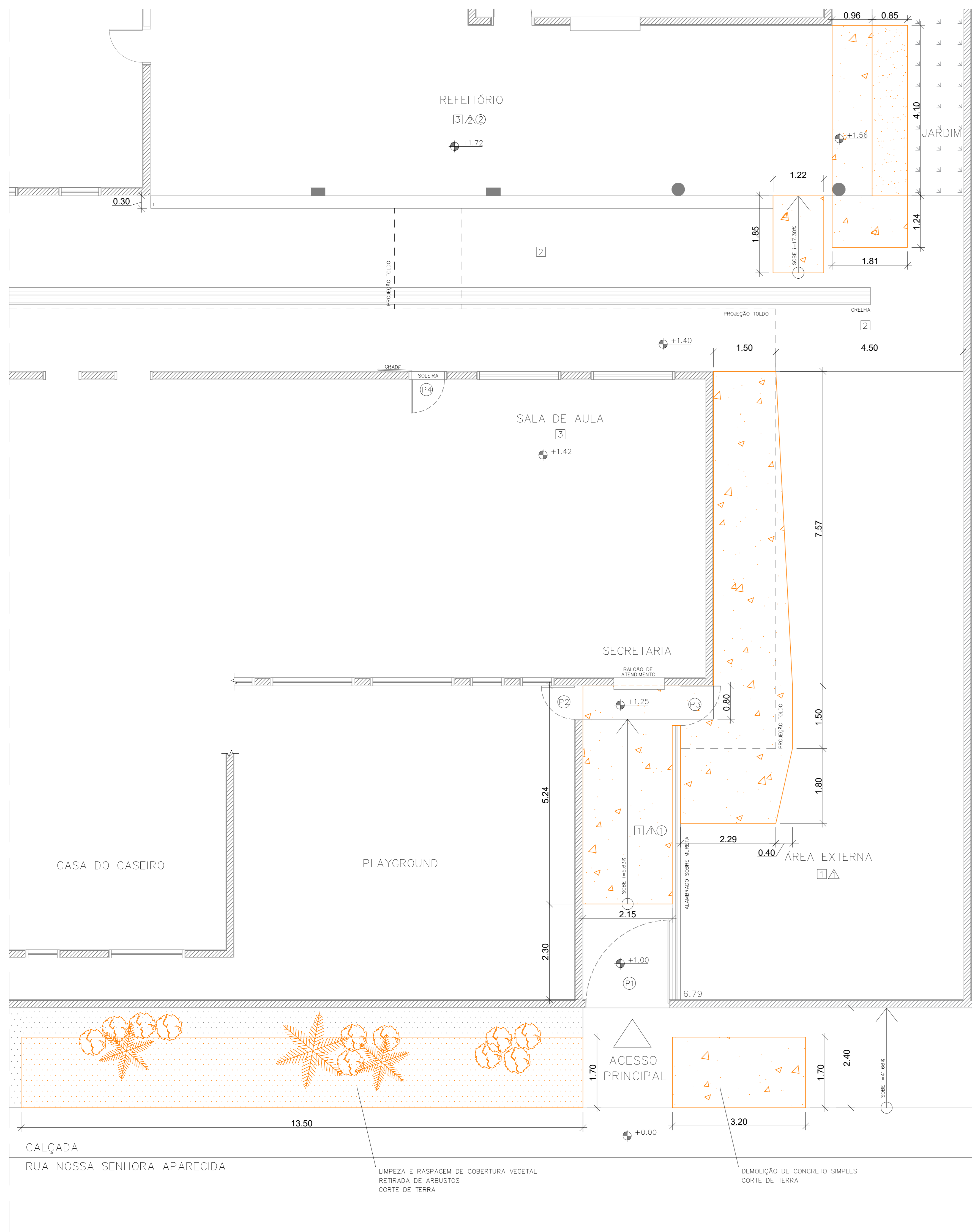
PLANTA DEMOLIÇÃO ESCALA 1:50
