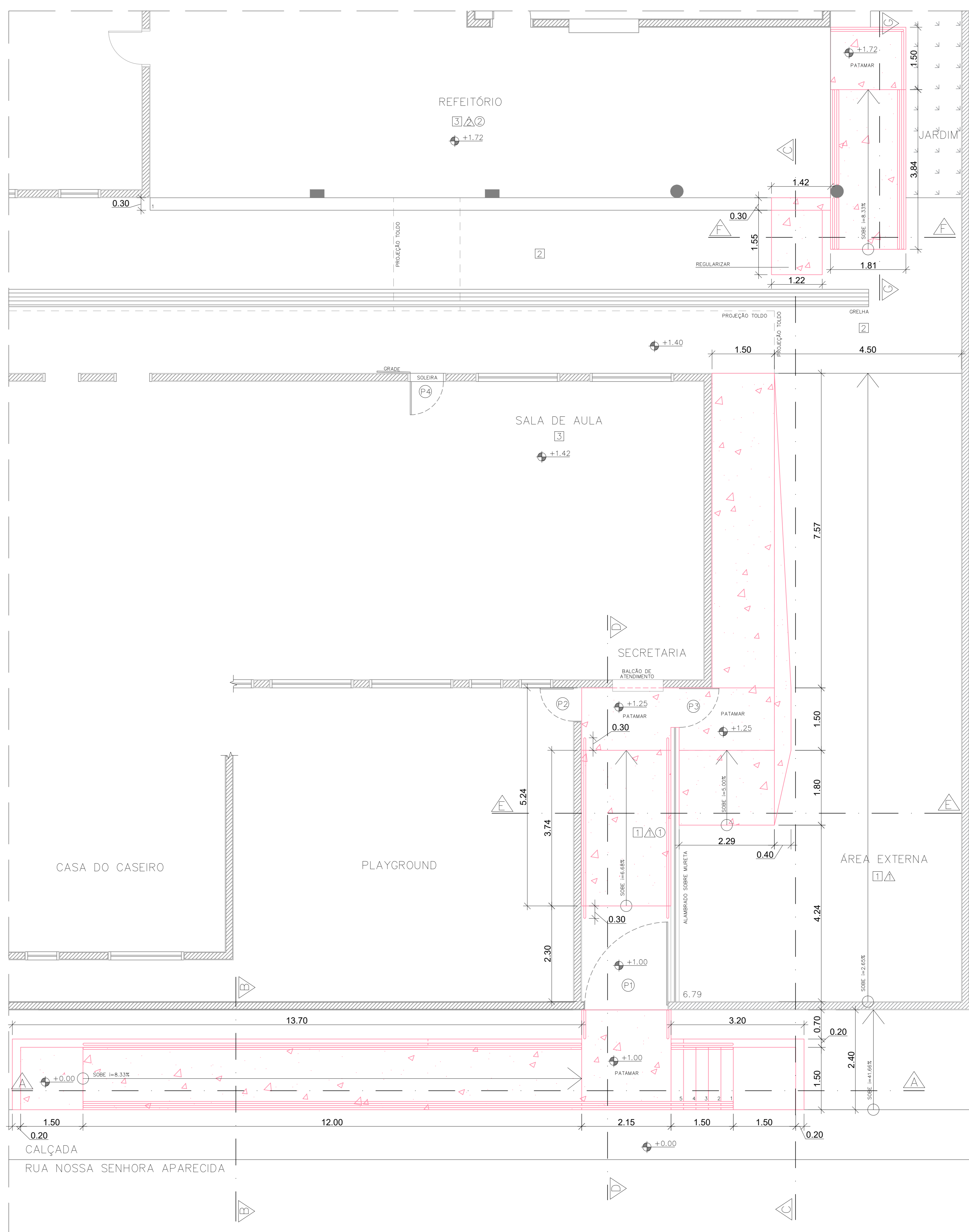
PLANTA CONSTRUÇÃO ESCALA 1:50
