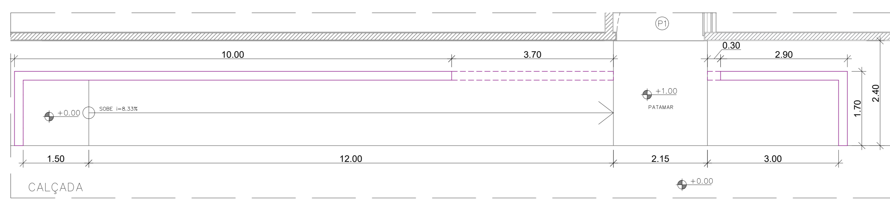
ESQUEMA MURO DE ARRIMO ESCALA 1:50
