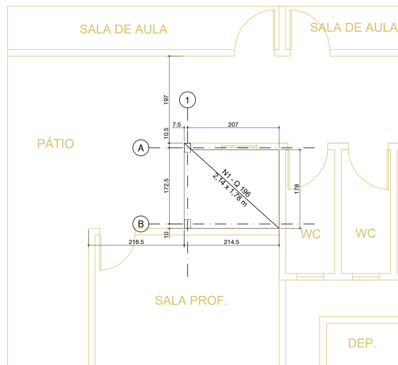
ARMAÇÃO RADIER COM TELA SOLDADA Q196 ESC.: 1:50
