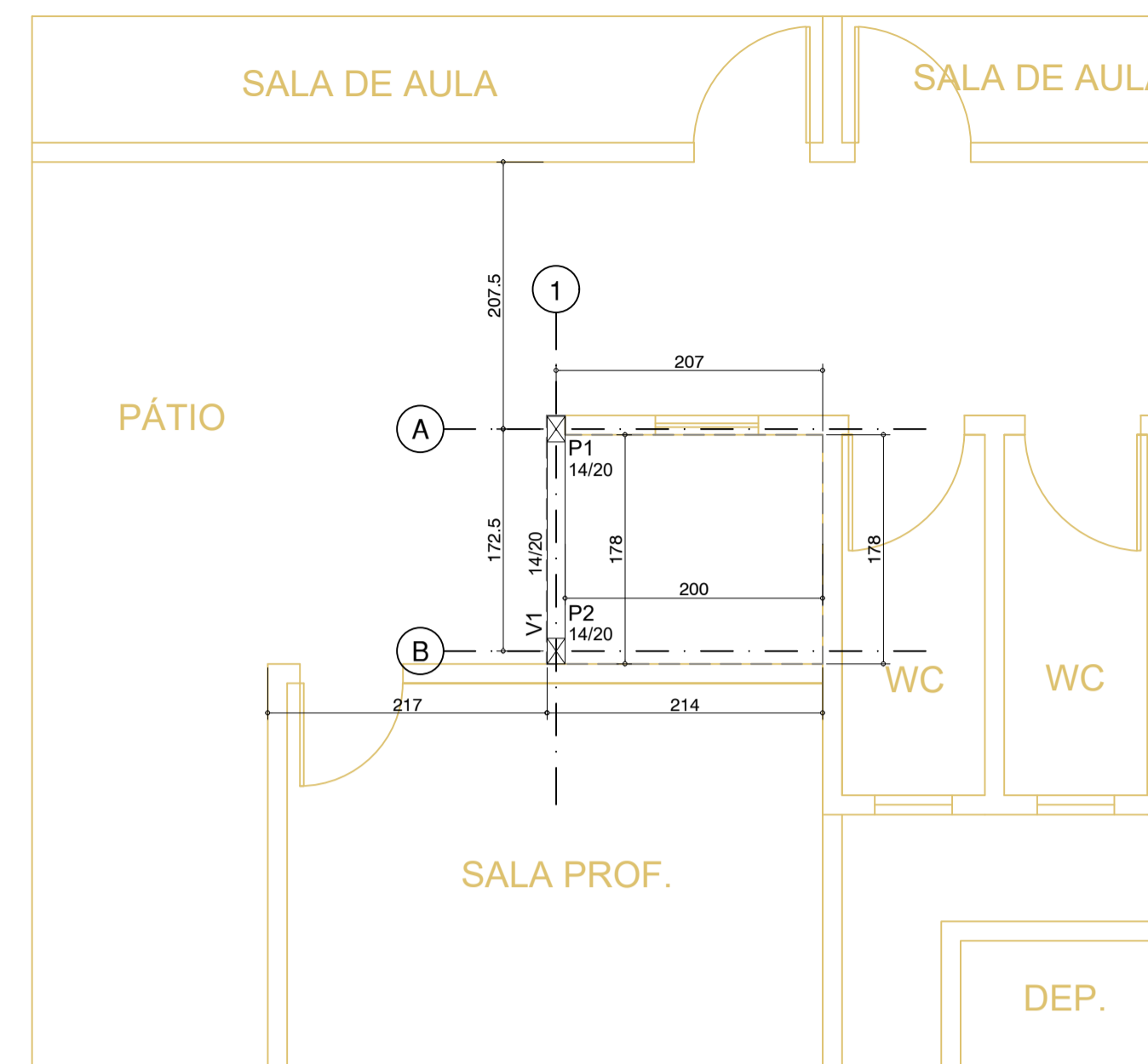
PLANTA DE FÔRMA COTA: +3,21m ESC.: 1:50
