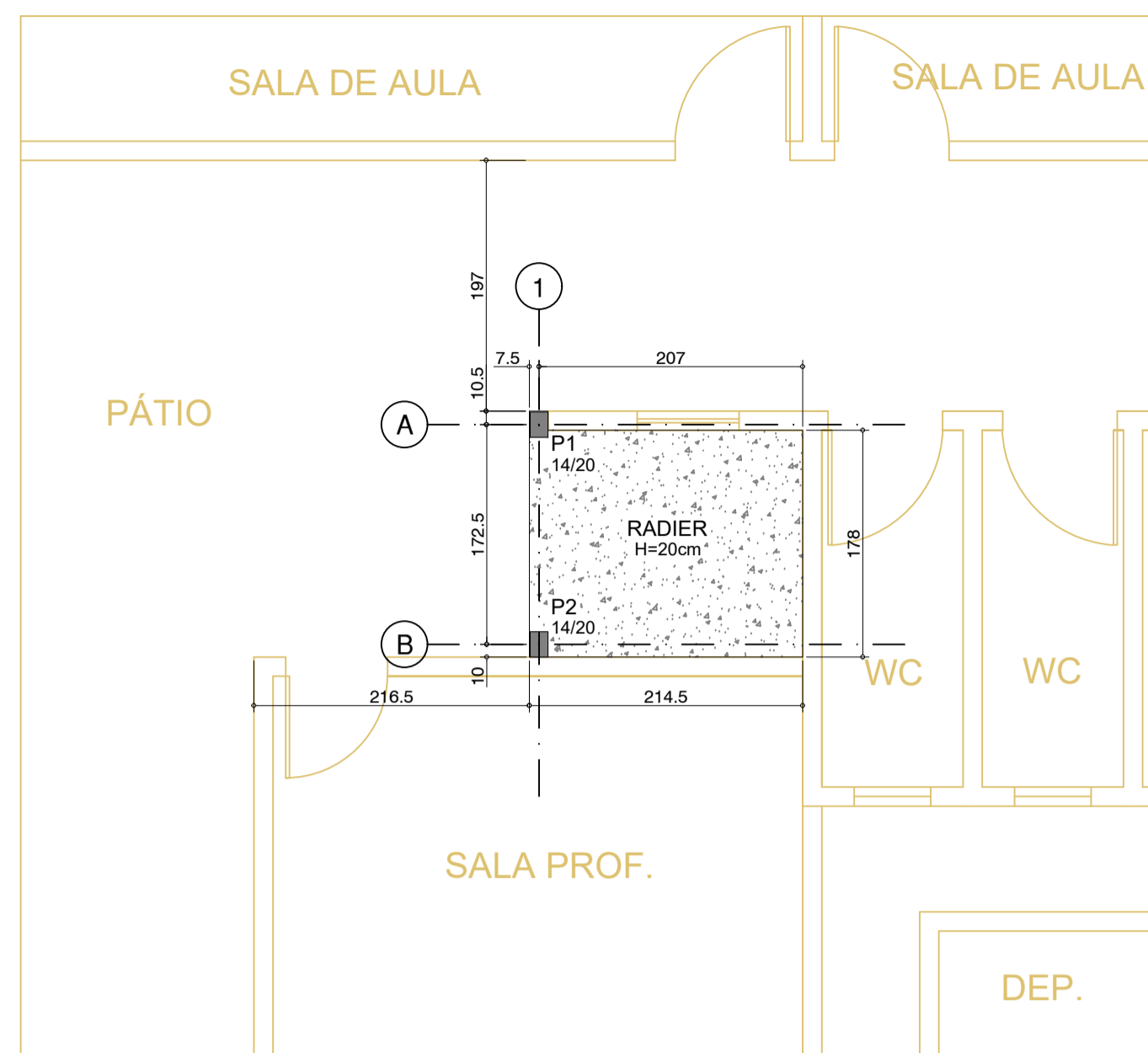
PLANTA DE FÔRMA LOCAÇÃO DE PILARES COTA: 0,00 ESC.: 1:50
