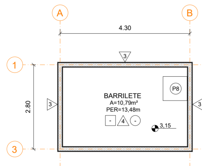
PLANTA DE BARRILETE ESC. 1:75
