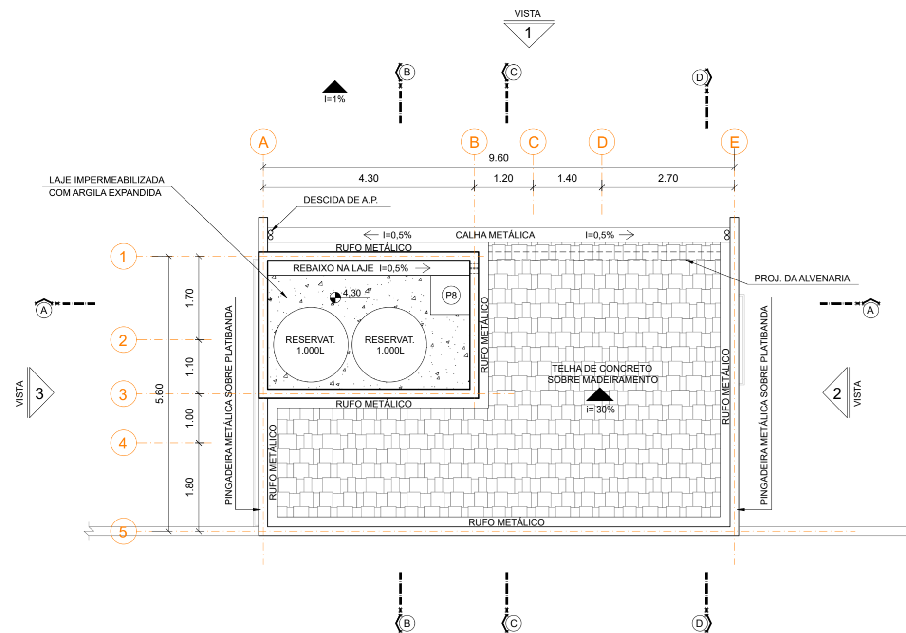
PLANTA DE COBERTURA ESC. 1:75
