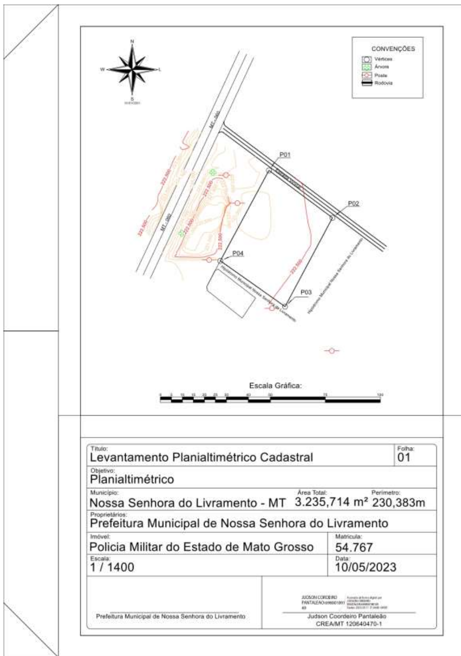
Figura 2: Levantamento Planialtimétrico Cadastral.
