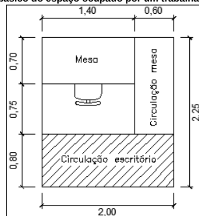
Figura 1 - Módulo básico do espaço ocupado por um trabalhador em escritório (m)
