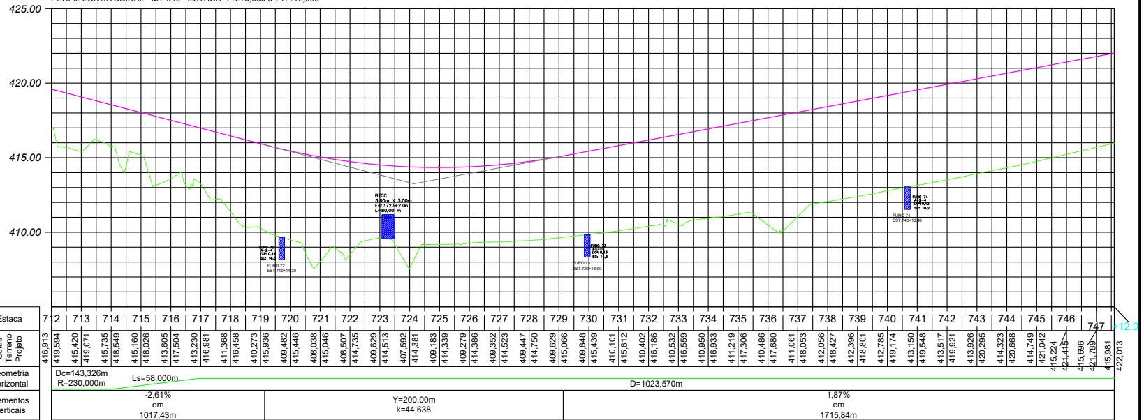
PERFIL LONGITUDINAL - MT-040 - ESTACA=712+0,000 à 747+12,000
