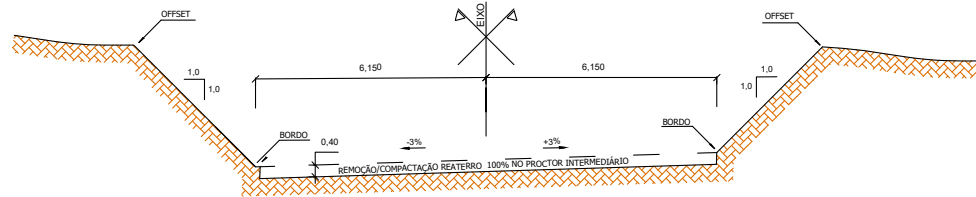
INTERSEÇÃO 01 - RÓTULA CORTE
