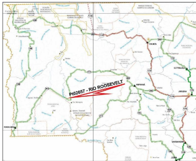
Mapa de Situação – Ponte sobre o Rio Roosevelt (PT02657).
