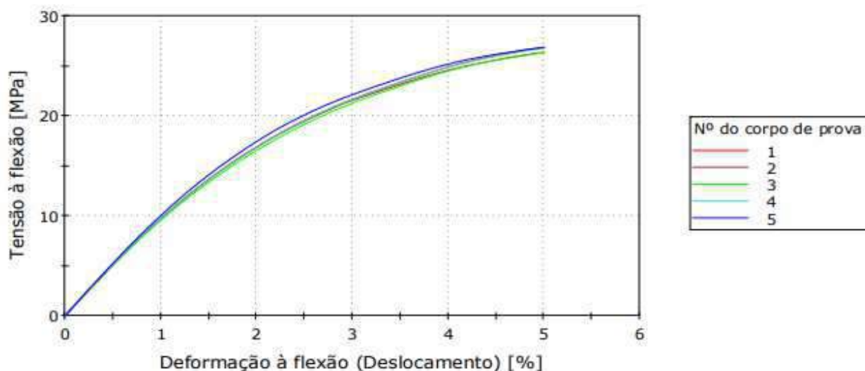
Figura 6 – Curvas Tensão x Deformação da amostra AFK246038.
