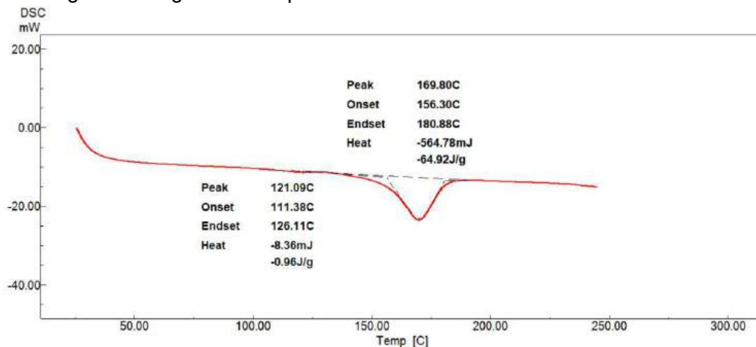
Figura 3 – Curva DSC da amostra AFK246038 – 1º Aquecimento.
