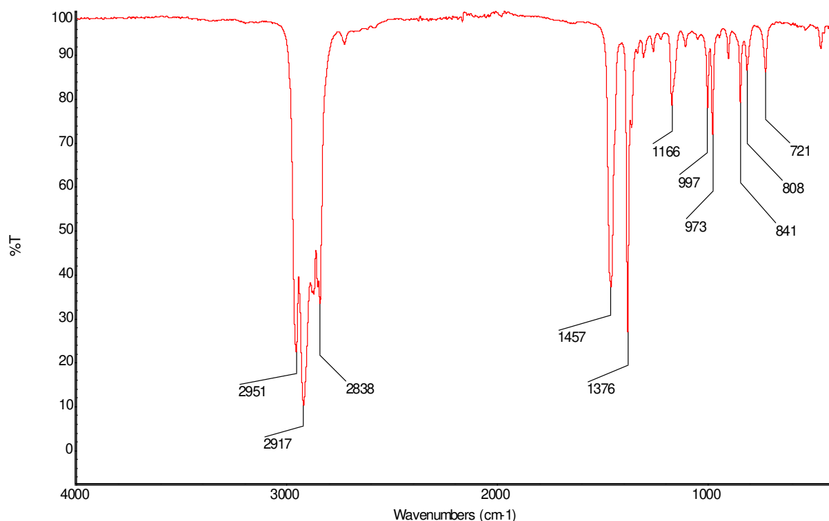
Figura 2 – Espectro no infravermelho da amostra AFK246038 (—).
