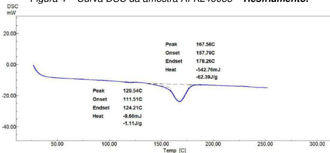
Figura 5 – Curva DSC da amostra AFK246038 – 2º Aquecimento.
