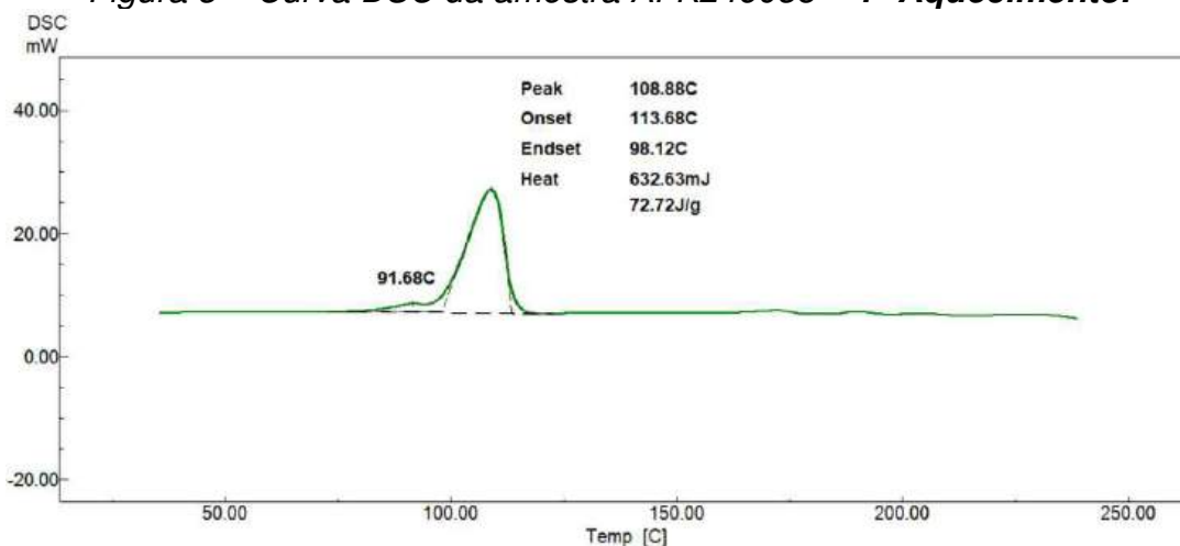
Figura 4 – Curva DSC da amostra AFK246038 – Resfriamento.
