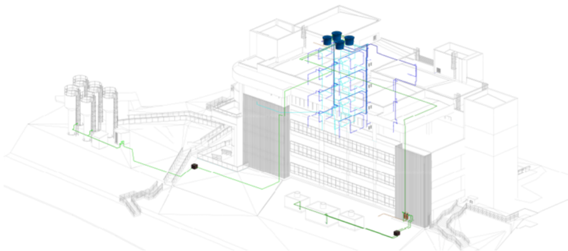
Isométrico implantação água fria
