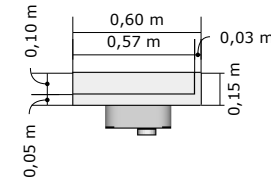
VISTA LATERAL- BANCADA
