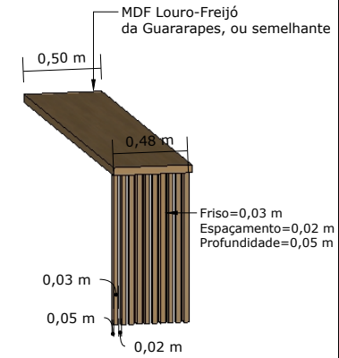
VISTA PERSPECTIVA - BANCADA ALTA
