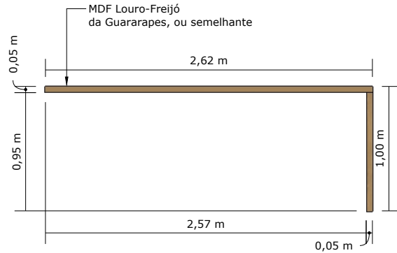
VISTA FRONTAL- BANCADA ALTA
