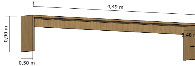
VISTA PERSPECTIVA - BANCADA ALTA DE TRABALHO
