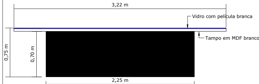
VISTA FRONTAL - MESA DE REUNIÃO
