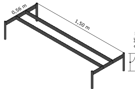
DETALHE EM PERSPECTIVA DA BASE DE METAL - "PÉ" DA FLOREIRA
