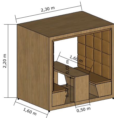
VISTA PERSPECTIVA 1 - CABINE MÓVEL
