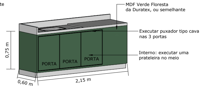
VISTA PERSPECTIVA - ARMÁRIO BANCADA
