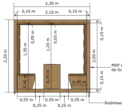
VISTA FRONTAL - CABINE MÓVEL
