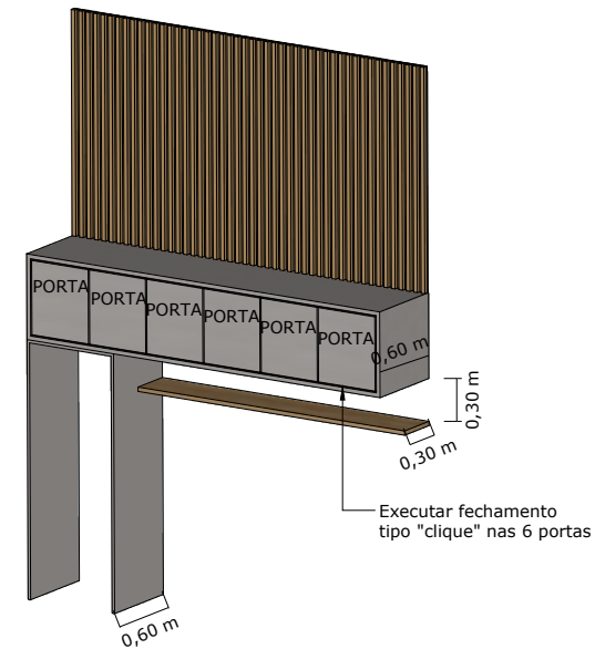
VISTA PERSPECTIVA - ARMÁRIO SUPERIOR, PRATELEIRA PAINEL RIPADO
