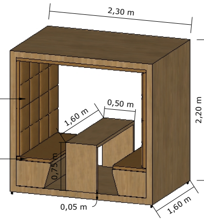
VISTA PERSPECTIVA 2 - CABINE MÓVEL
