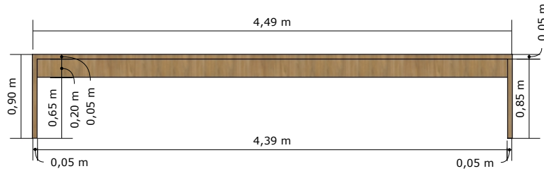
VISTA FRONTAL - BANCADA ALTA DE TRABALHO
