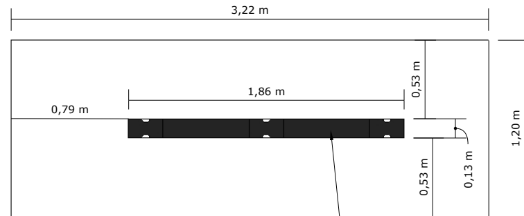
VISTA SUPERIOR- MESA DE REUNIÃO
