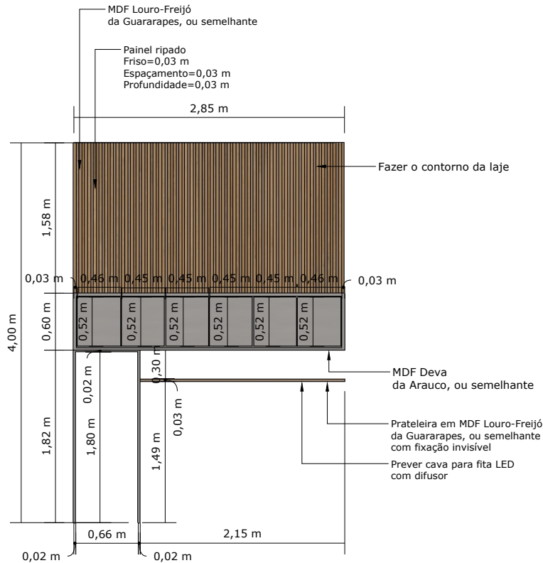
VISTA FRONTAL - ARMÁRIO SUPERIOR, PRATELEIRA PAINEL RIPADO
