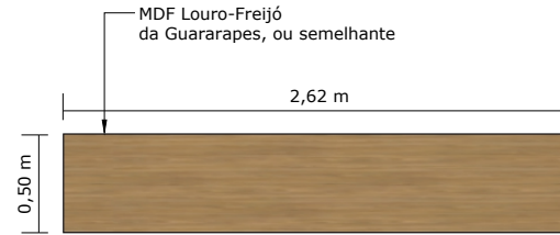
VISTA SUPERIOR- BANCADA ALTA
