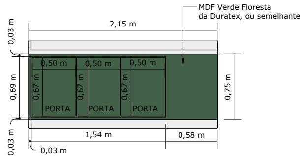
VISTA FRONTAL- ARMÁRIO BANCADA
