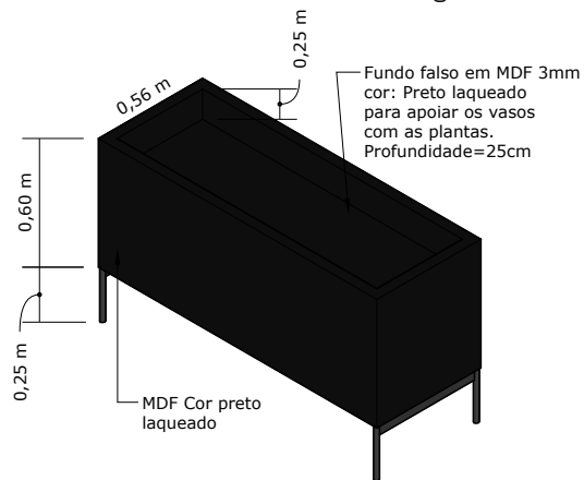
VISTA PERSPECTIVA SEM PLANTAS - FLOREIRA
