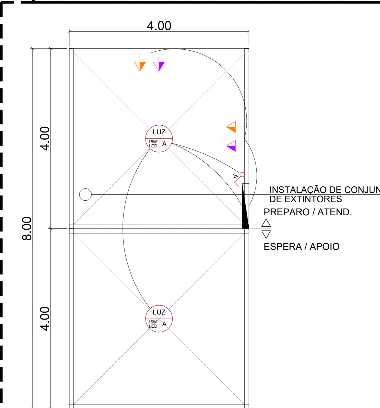
BARRACA - TIPO 1 ESCALA 1:50
