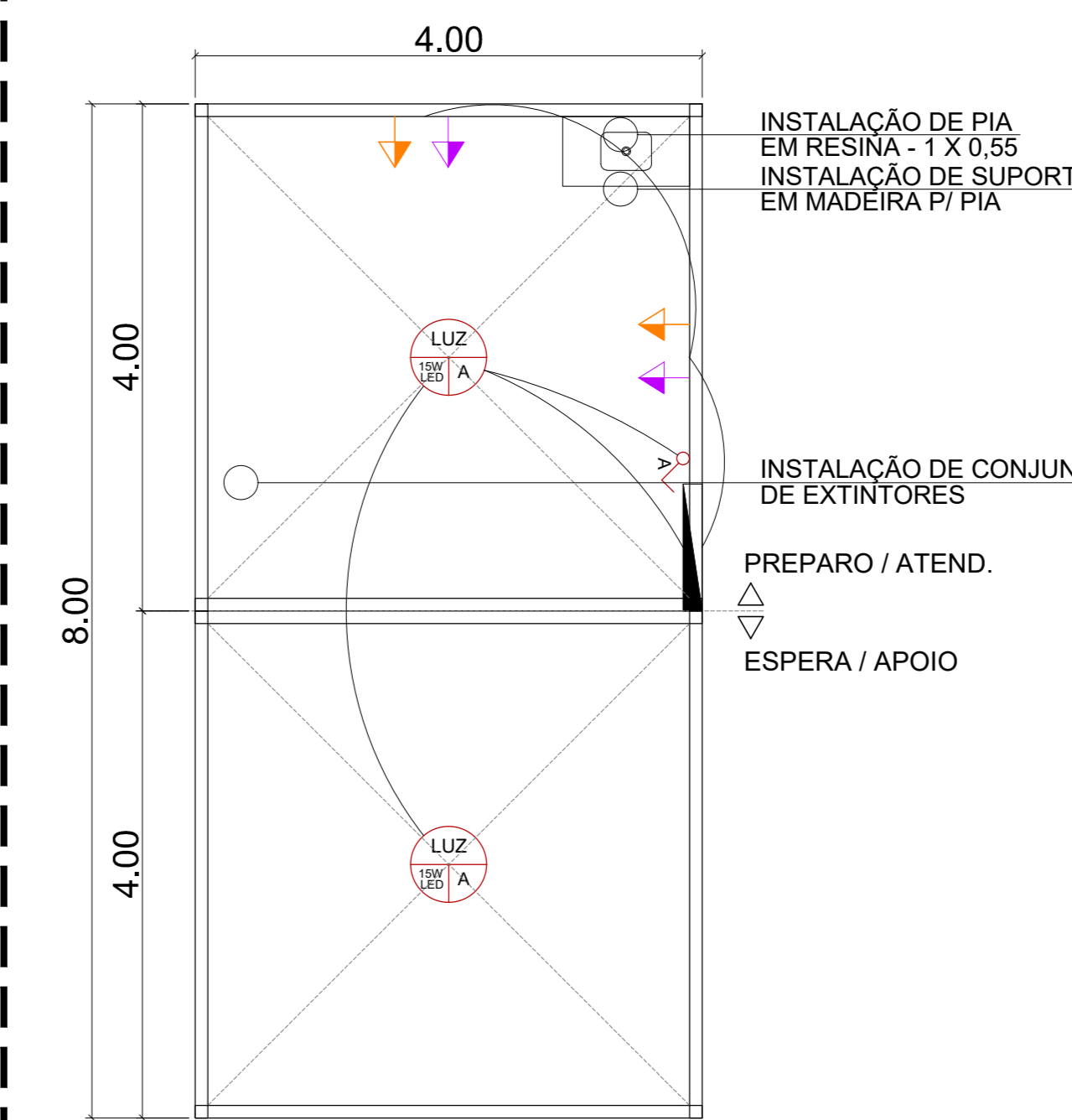
BARRACA - TIPO 2 ESCALA 1:50
