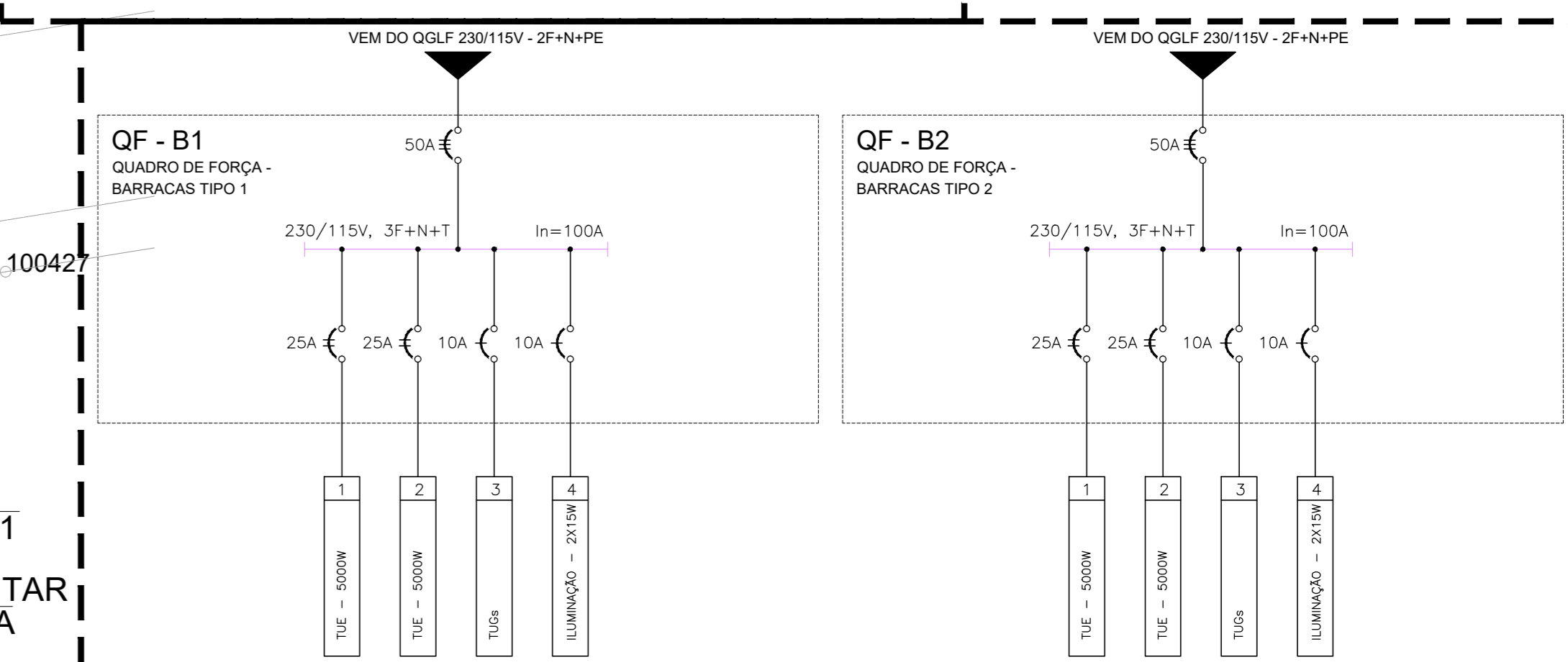
DIAGRAMA UNIFILAR GERAL
