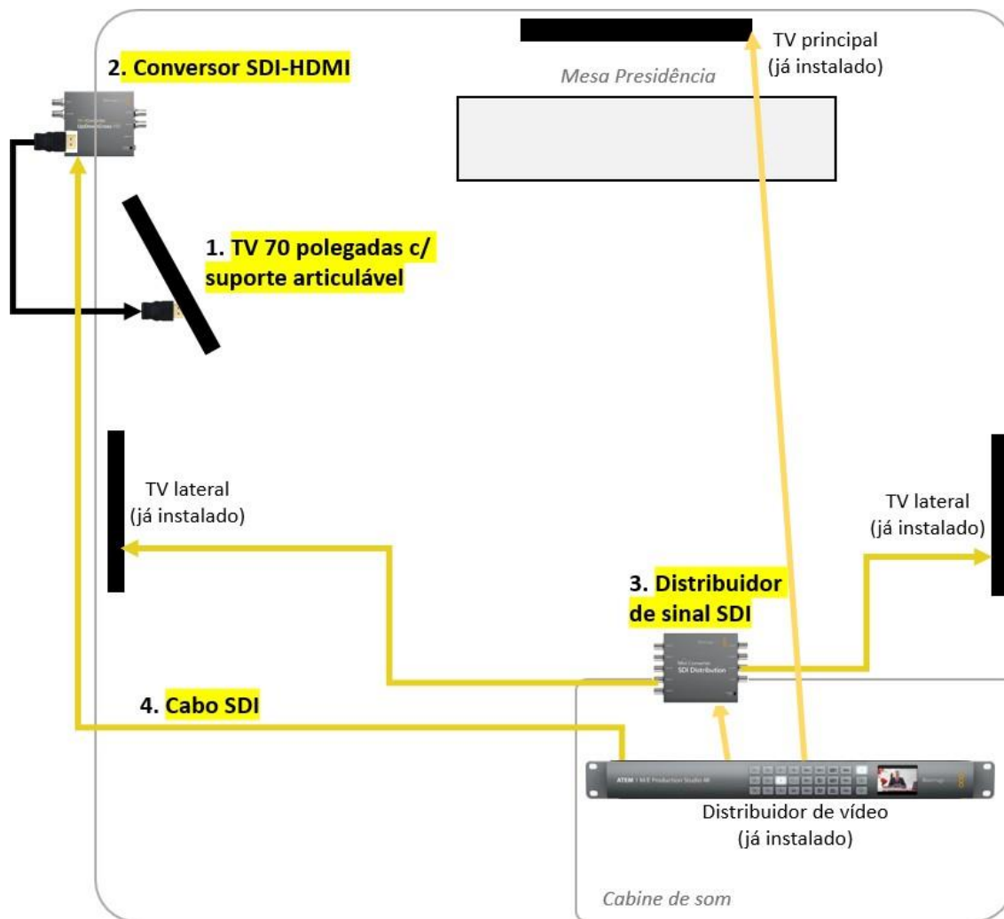
Esquema de ligação do novo sistema de vídeo
