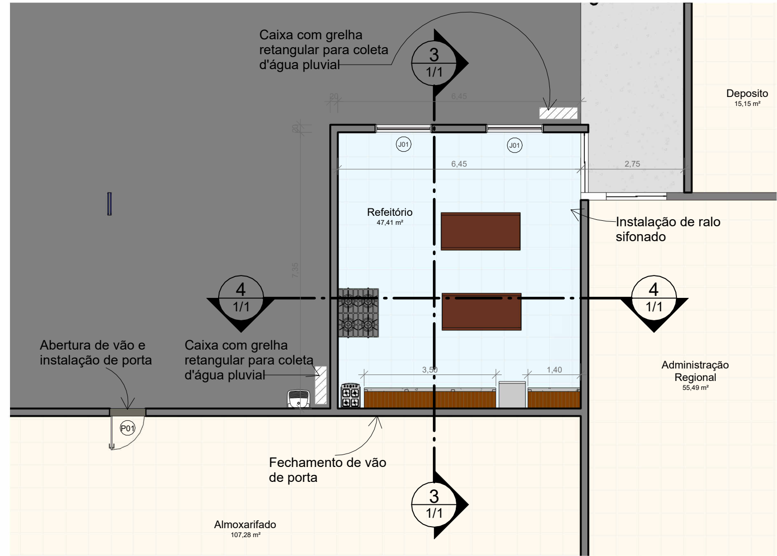
2 TÉRREO ESCALA 1 : 100
