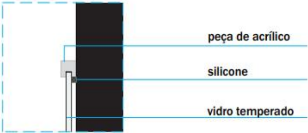
Vitrine Vertical - Elevação Lateral Det.
