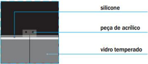
Vitrine Vertical - Elevação Frontal Det.
