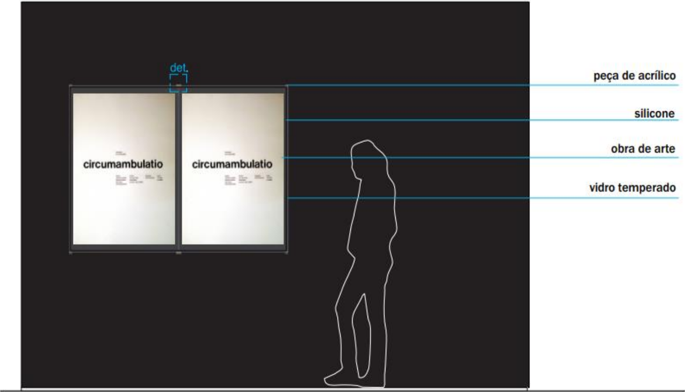
Vitrine Vertical - Elevação Frontal
