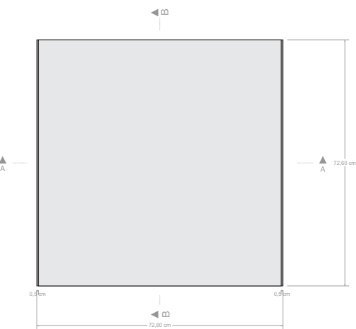
VISTA INFERIOR TAMPO EM ACRÍLICO LEITOSO 5mm
