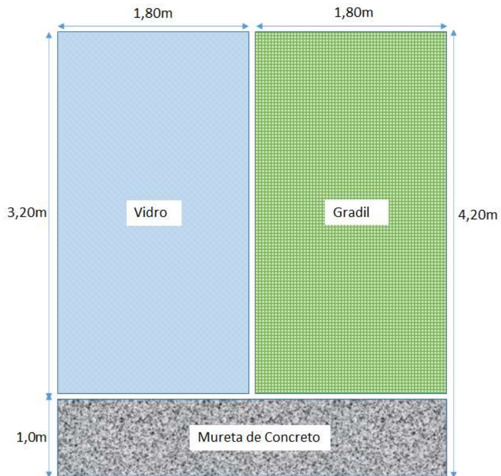
Figura 2 – Medidas do muro de vidro e gradis
