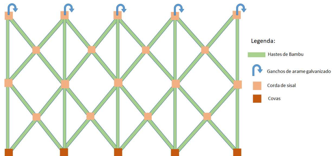
1B – Esquema de montagem das tramas de bambu
