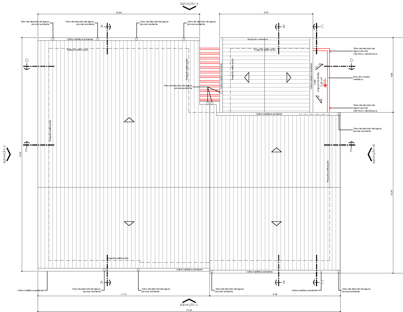
PLANTA COBERTURA Escala 1:75
