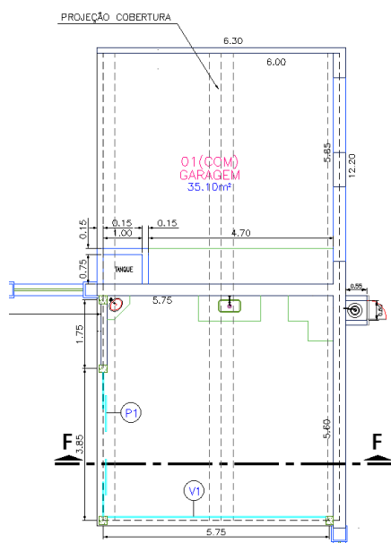
Figura 7 – Anexo 02 pós reforma
