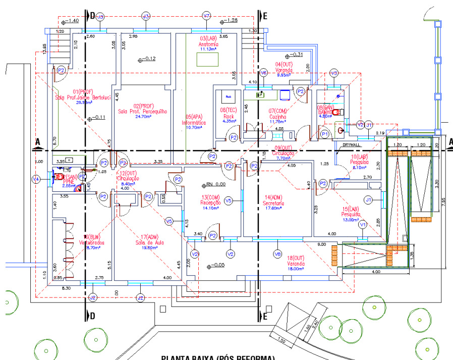
PIANTA RAÍZA (PÓS REFORMA) Figura 5 – Casa principal pós reforma
