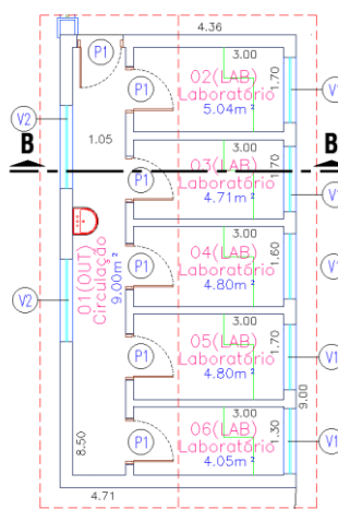
Figura 8 – Anexo 03 pós reforma
