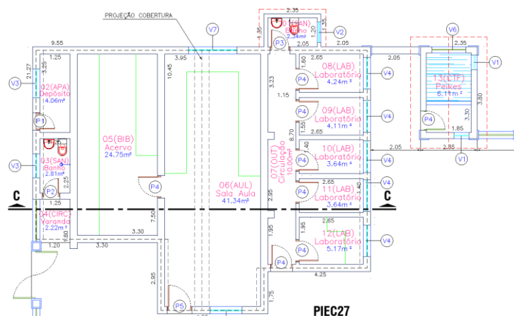
Figura 6 – Anexo 01 pós reforma
