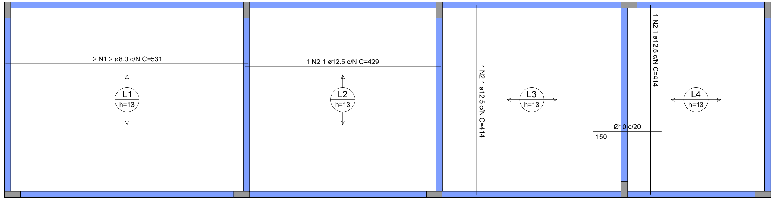
ARMAÇÃO POSITIVA E NEGATIVA DAS LAJES DO PAVIMENTO SUPERIOR 300
