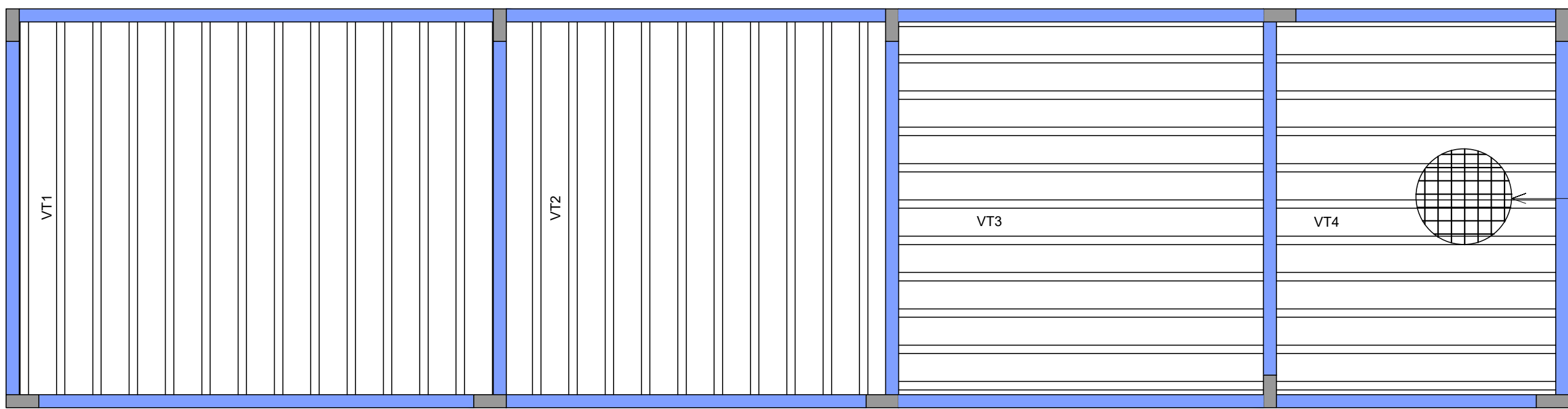
PLANTA DE VIGOTAS PRÉ-MOLDADAS
