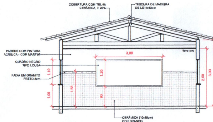
3 VISTA 1
