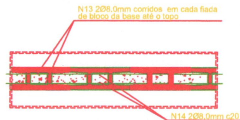
Detalhe 01 - planta baixa de 1 fiada de blocos estruturais
