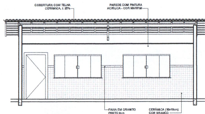
4 VISTA 2
