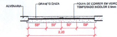
5 DET. JANELA01
