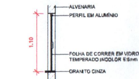
6 DET. JANELA01
