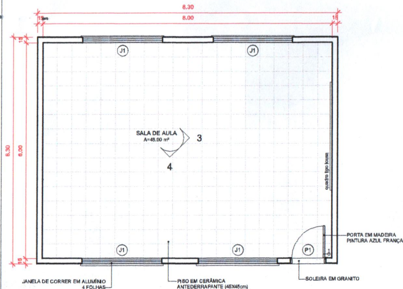
1 PLANTA BAIXA
