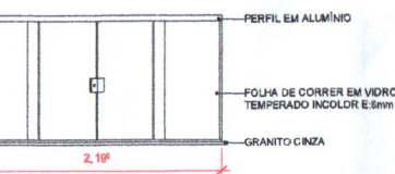
6 DET. JANELA01
