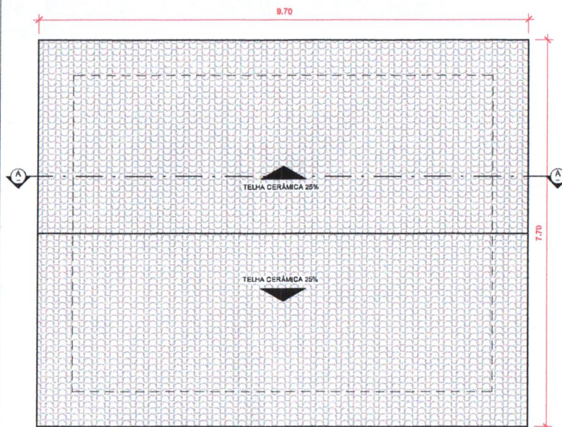
2 COBERTURA
