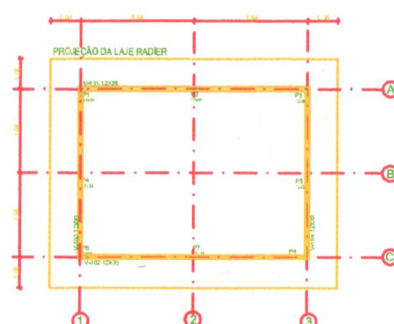
PLANTA DE VIGAMENTO
