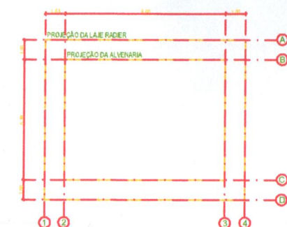
PLANTA DE LOCAÇÃO RADIER
