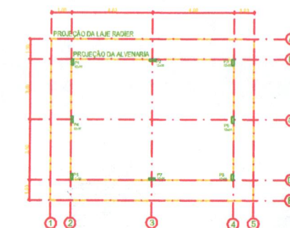
PLANTA DE LOCAÇÃO DE PILARES
