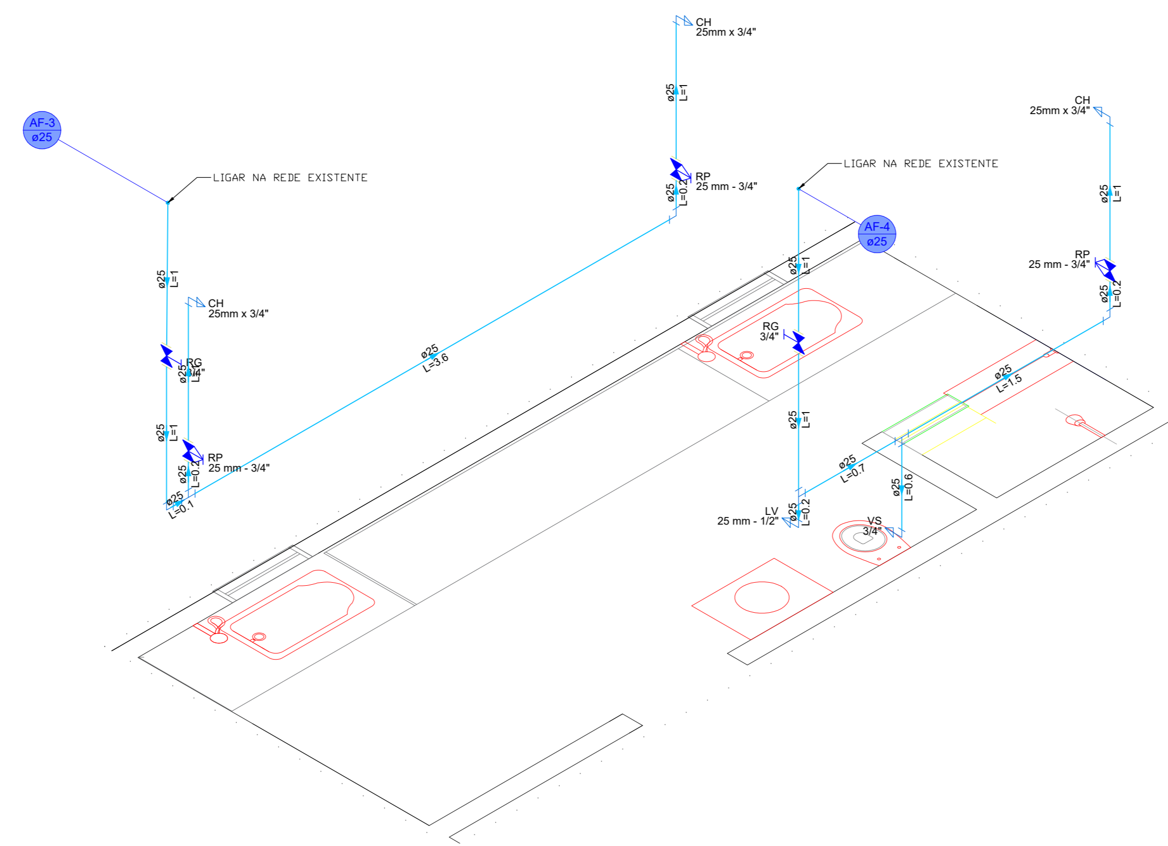
DETALHE HID-2 1:25
