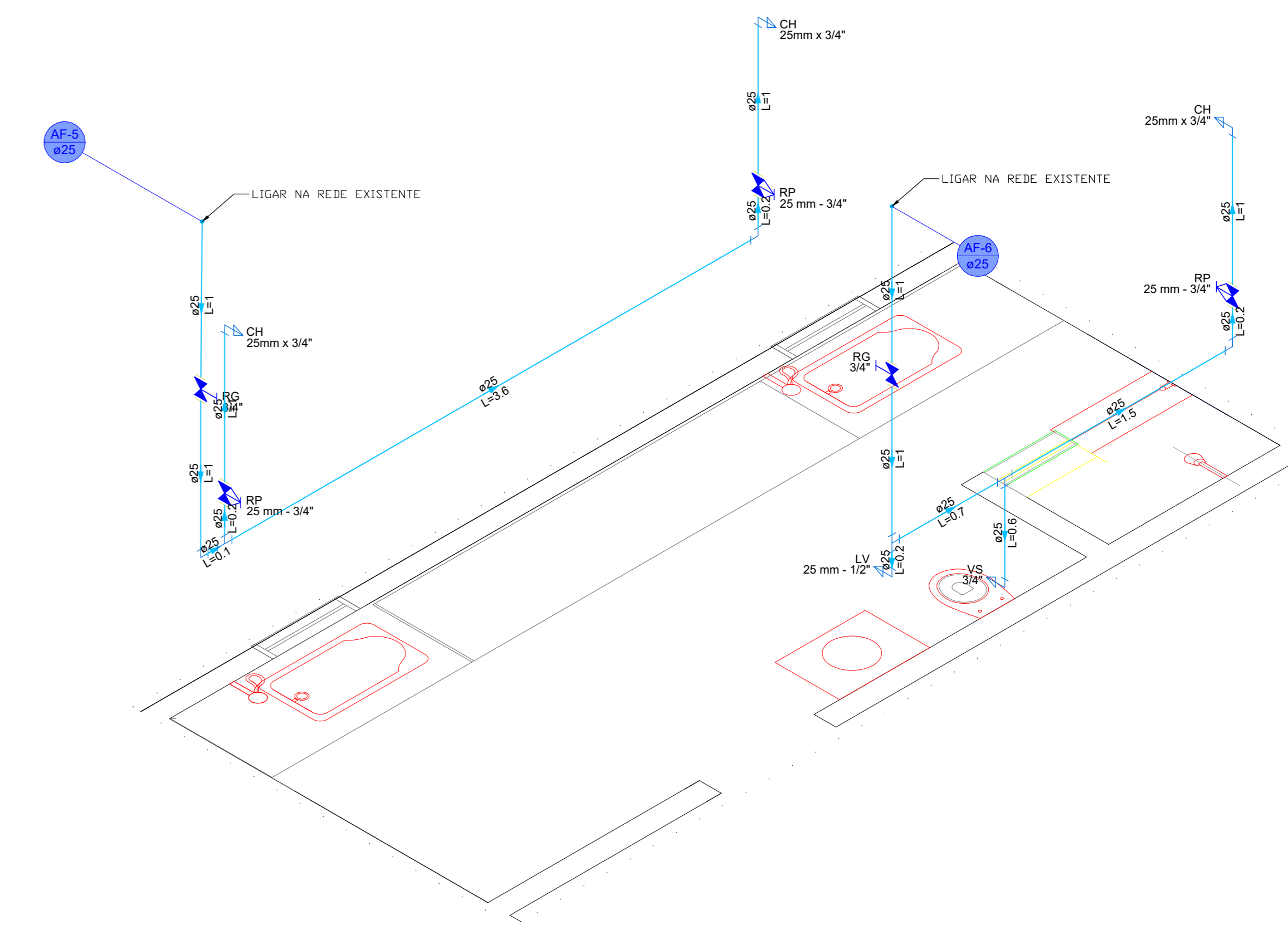
DETALHE HID-3 1:25
