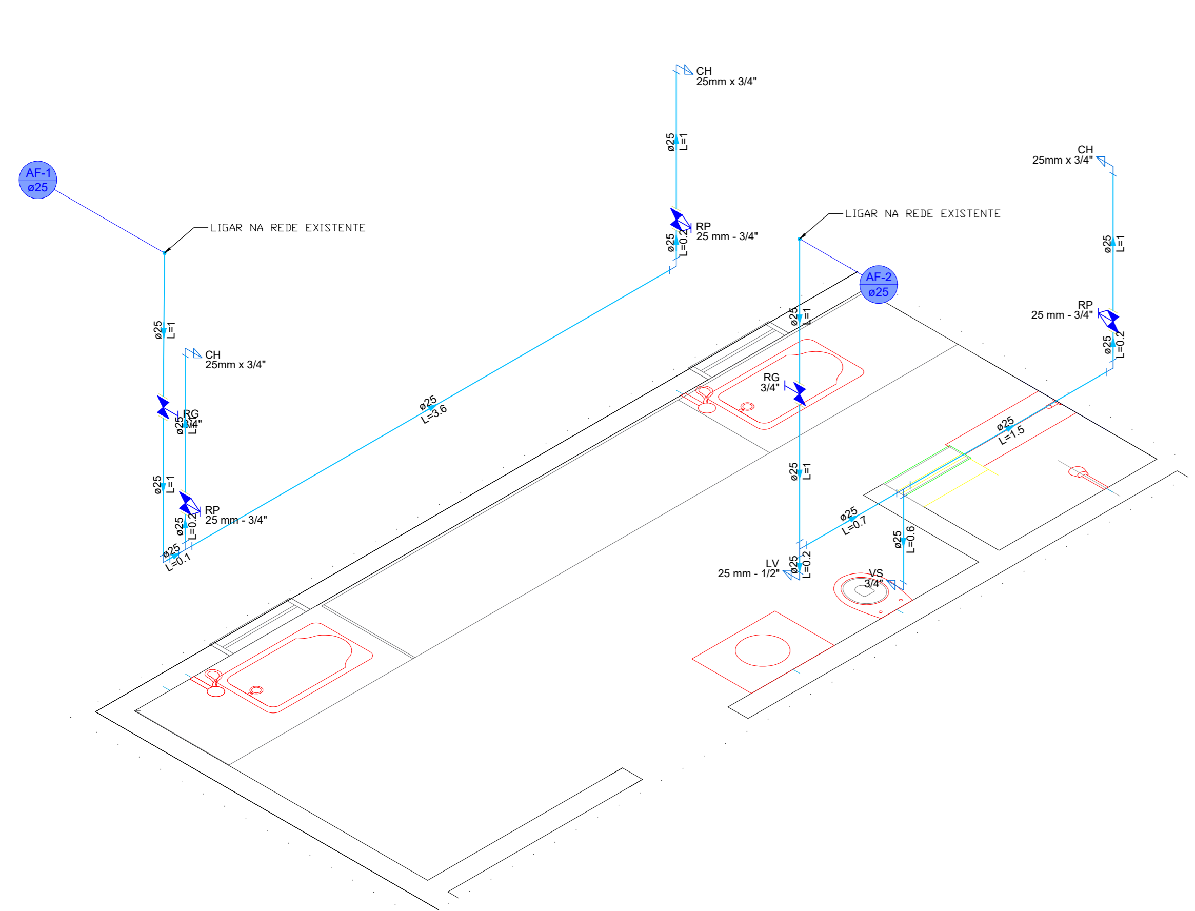
DETALHE HID-1 1:25
