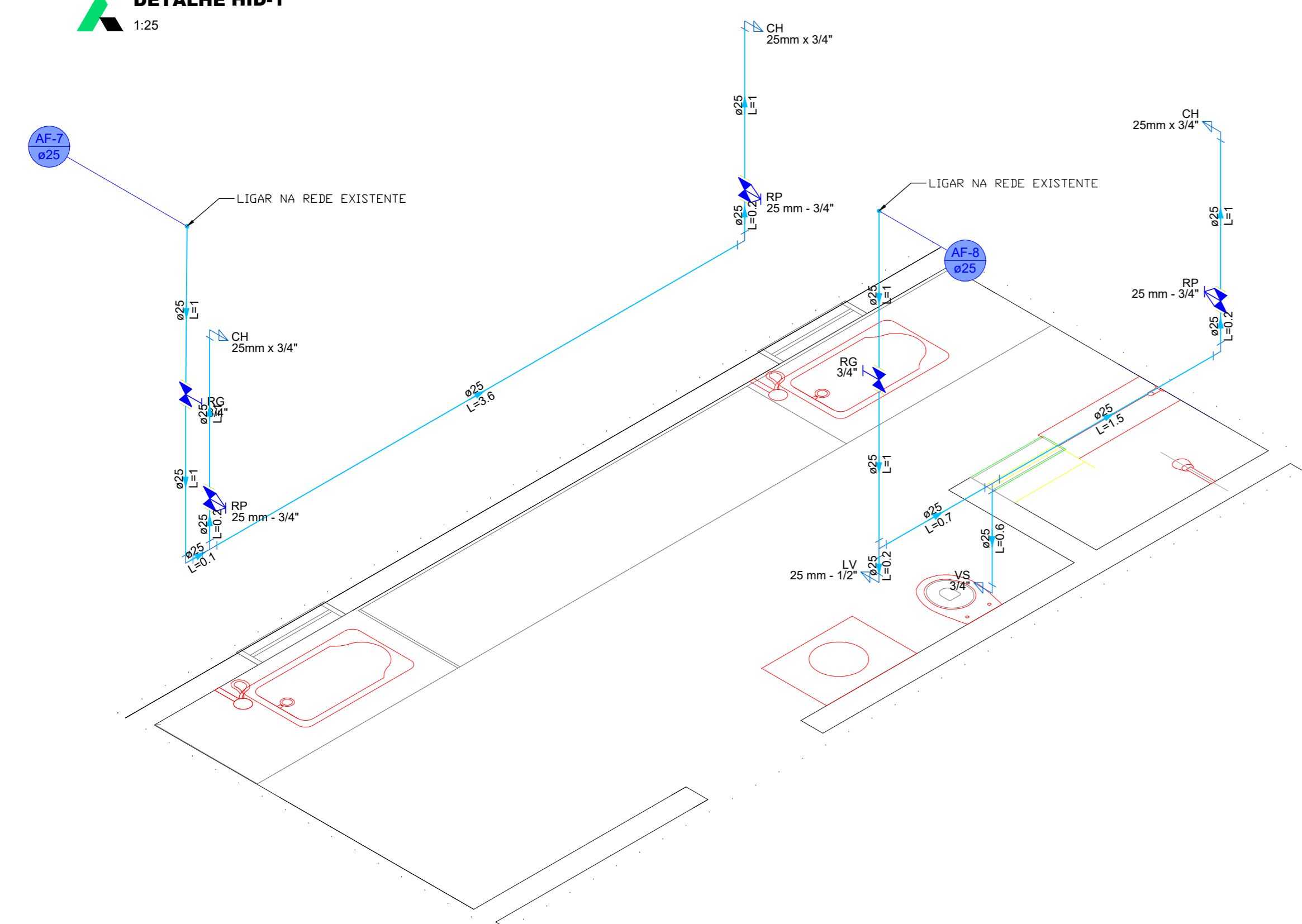
DETALHE HID-4 1:25
