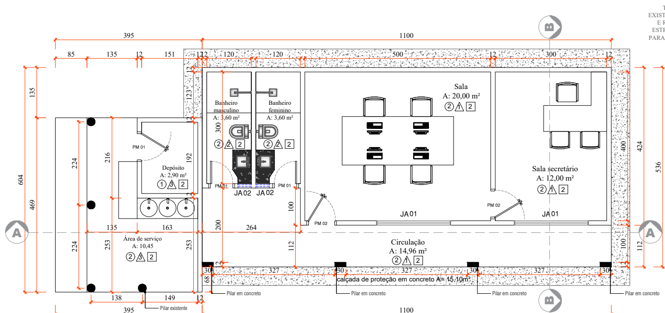
PLANTA BAIXA-GERAL-REFORMA E AMPLIAÇÃO
