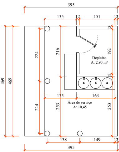
PLANTA BAIXA-EDIFICAÇÃO EXISTENTE
