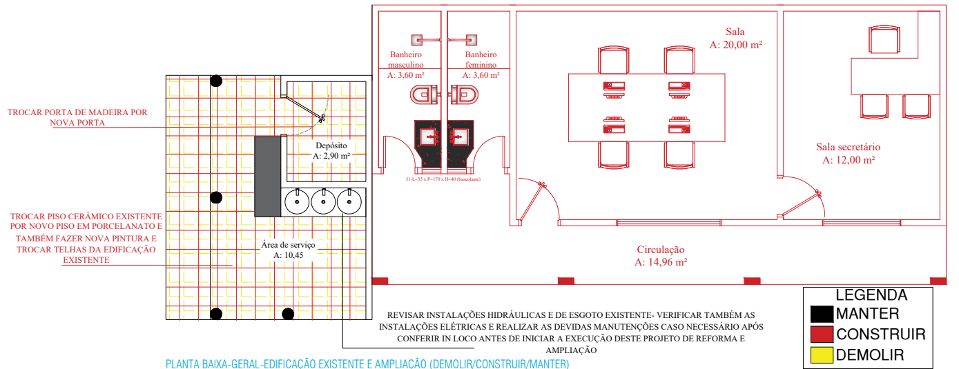
PLANTA BAIXA-GERAL-EDIFICAÇÃO EXISTENTE E AMPLIAÇÃO (DEMOLIR/CONSTRUIR/MANTER)
