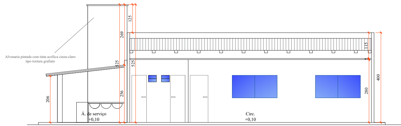
CORTE AA-REFORMA E AMPLIAÇÃO
