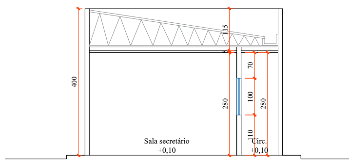
CORTE BB-REFORMA E AMPLIAÇÃO
