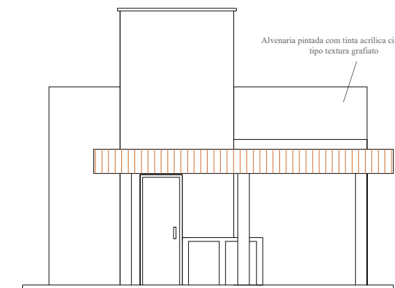
FACHADA LATERAL-REFORMA E AMPLIAÇÃO
