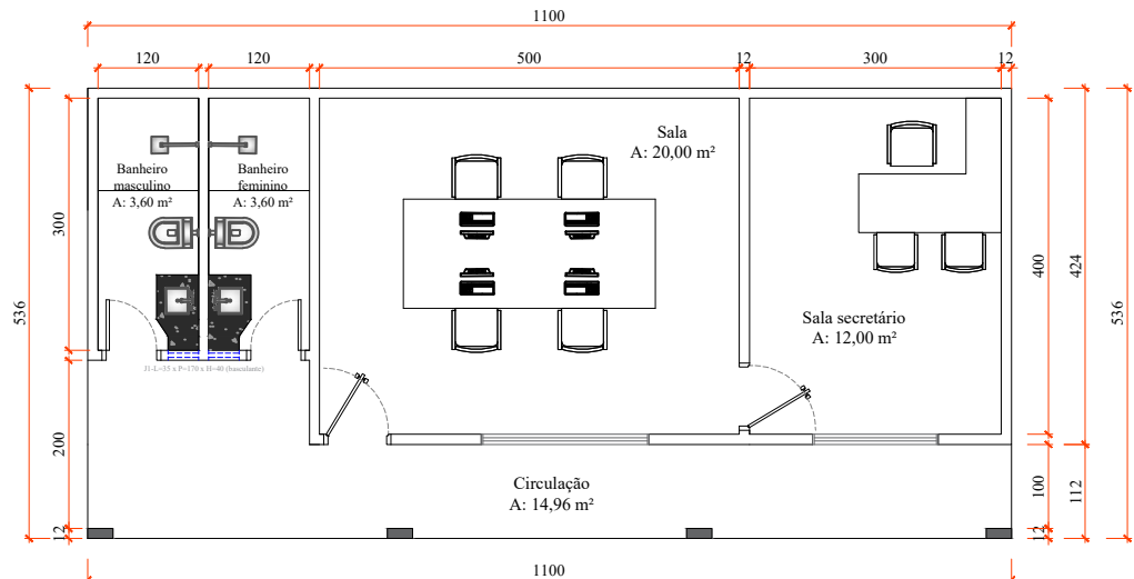
PLANTA BAIXA-AMPLIAÇÃO
