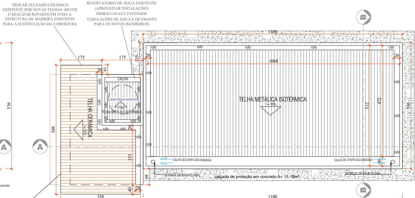
PLANTA DE COBERTURA-REFORMA E AMPLIAÇÃO
