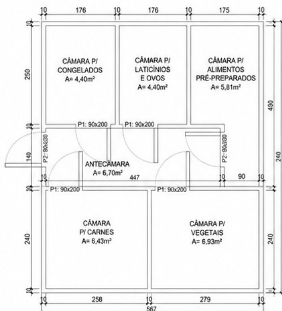
DETALHAMENTO - CÂMARA FRIGORÍFICA MODULAR SEM ESCALA
