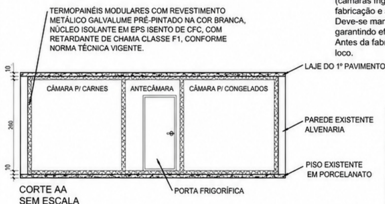
DETALHAMENTO - CÂMARA FRIGORÍFICA MODULAR SEM ESCALA
