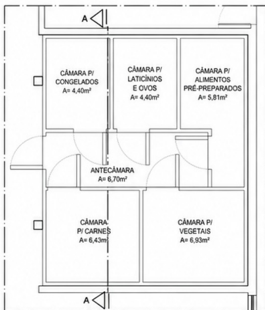
PLANTA BAIXA - CÂMARA FRIGORÍFICA MODULAR SEM ESCALA
