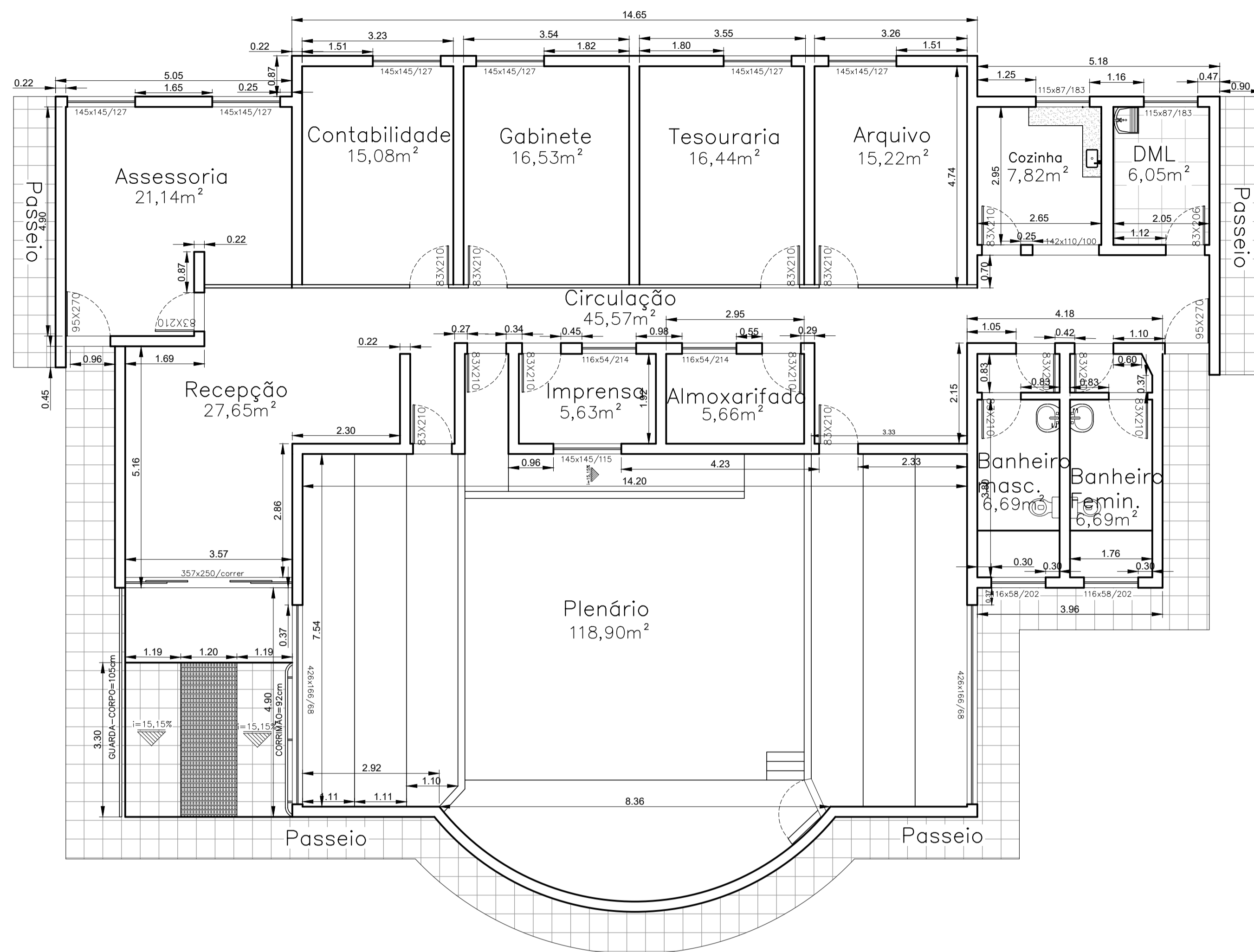
PLANTA BAIXA - (LEVANTAMENTO ARQUITETÔNICO) ESCALA: 1/75 (ÁREA:351,09m²)
