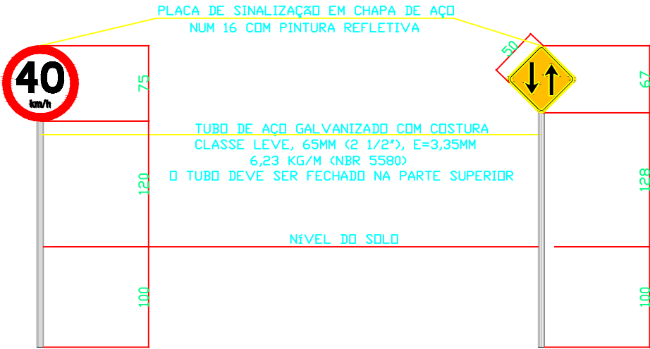
DETALHE DE SINALIZAÇÃO ESCALA= 1:50
