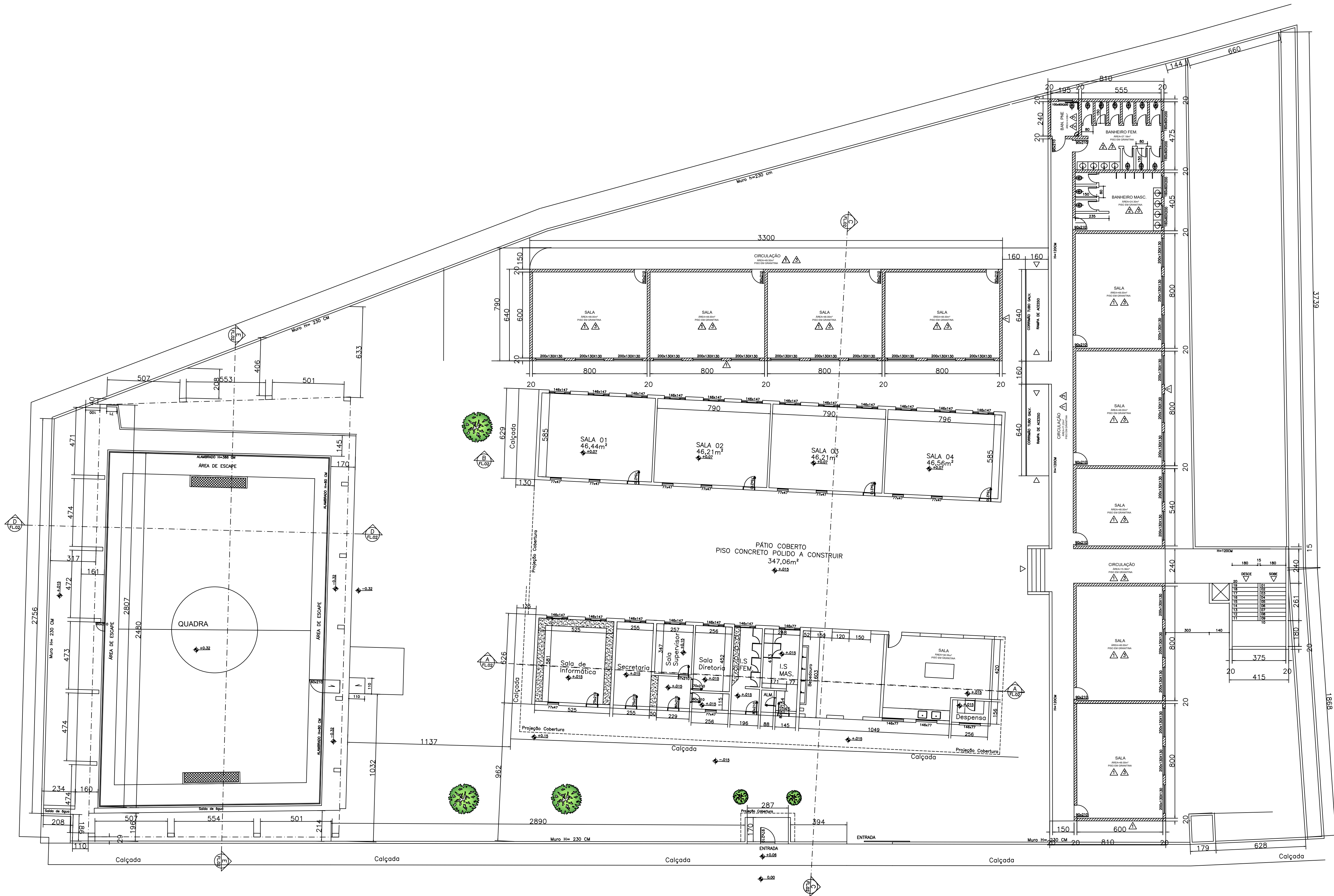
PLANTA BAIXA ESC. 1:150
