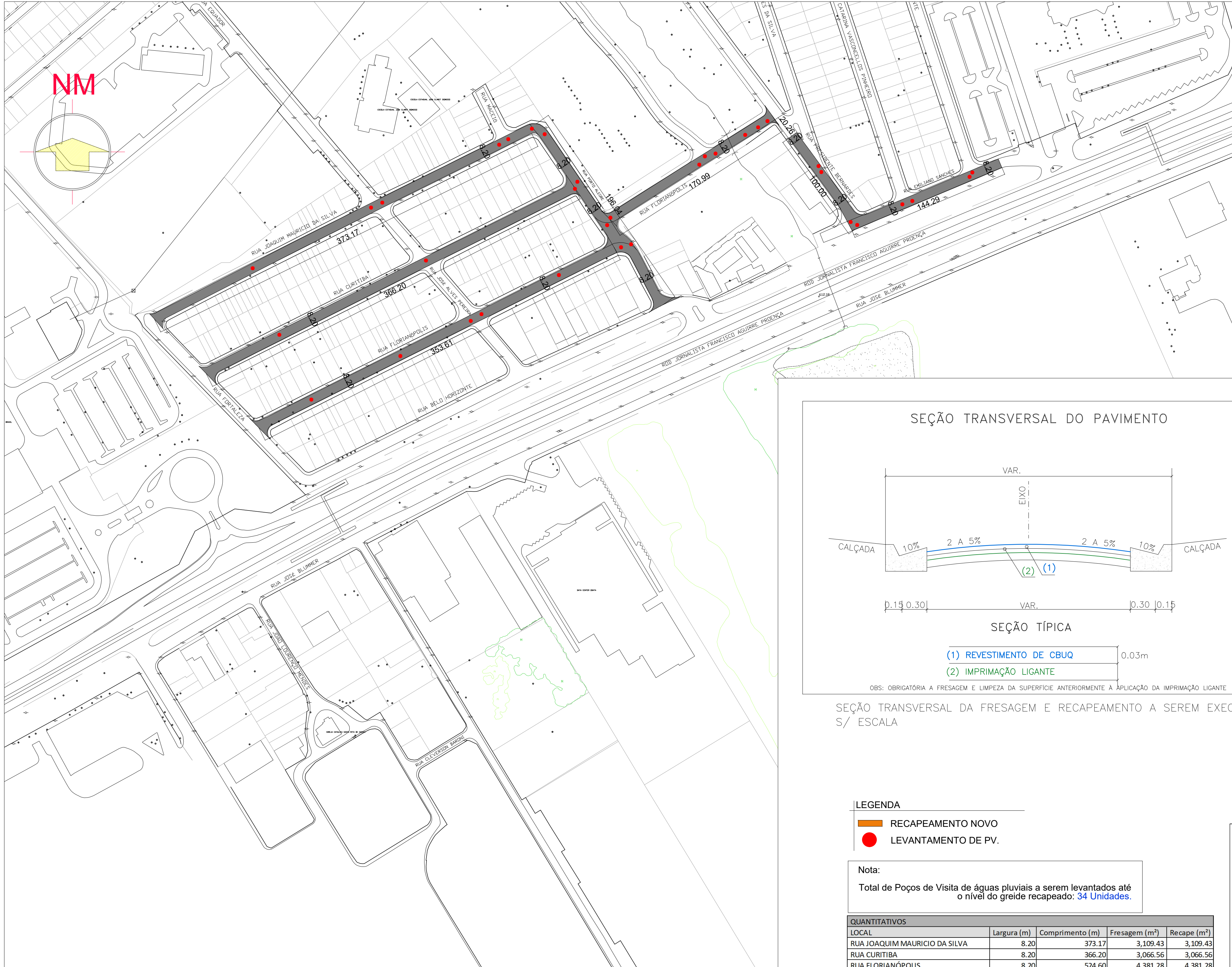
PLANTA GERAL DAS RUAS A SEREM RECAPEADAS ESC: 1:2.000
