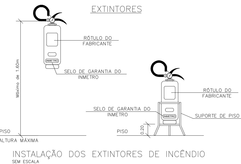
INSTALAÇÃO DOS EXTINTORES DE INCÊNDIO SEM ESCALA
