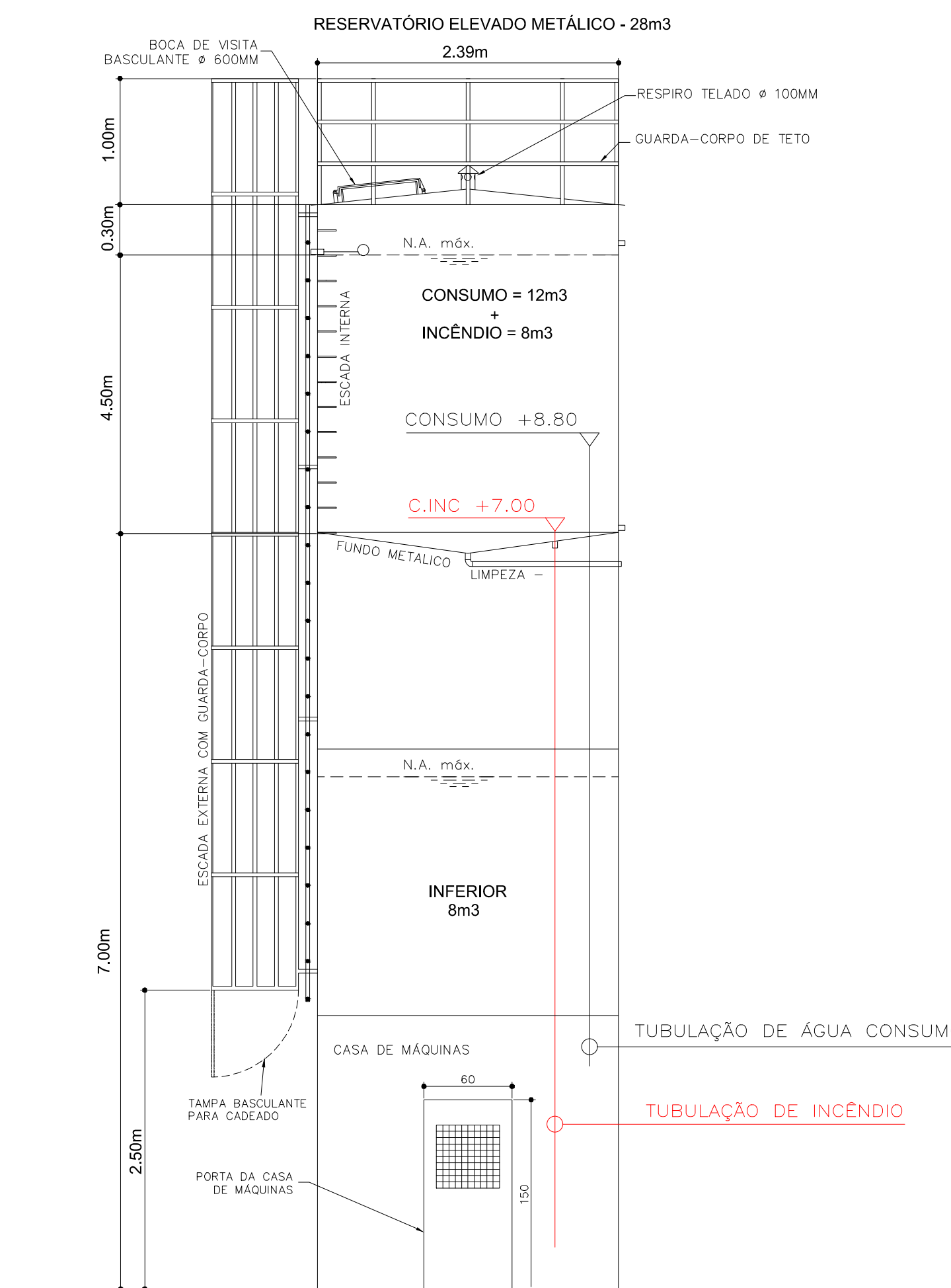
RESERVATÓRIO ELEVADO - 23.000 LITROS SEM ESCALA
