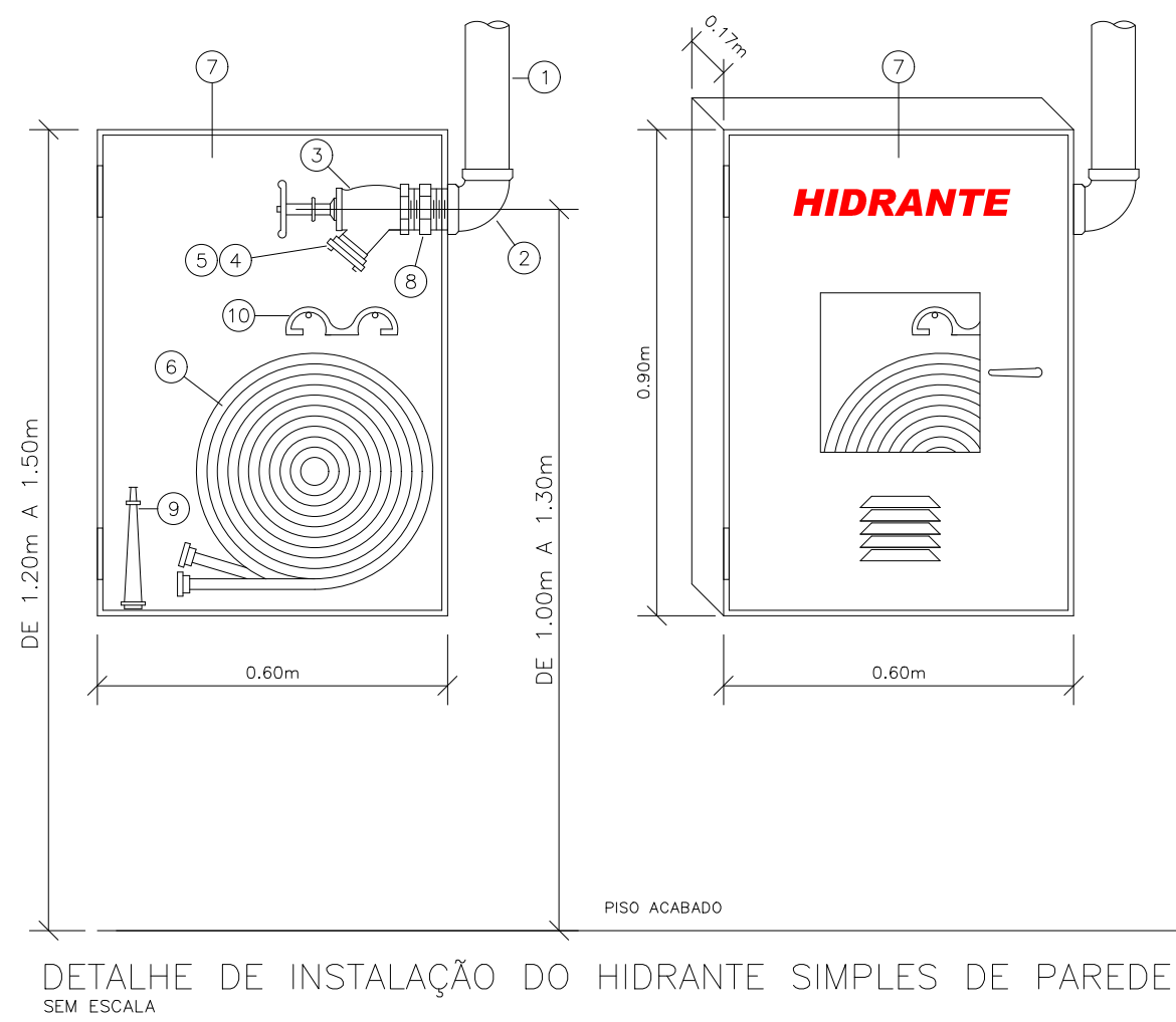
DETALHE DE INSTALAÇÃO DO HIDRANTE SIMPLES DE PAREDE SEM ESCALA
