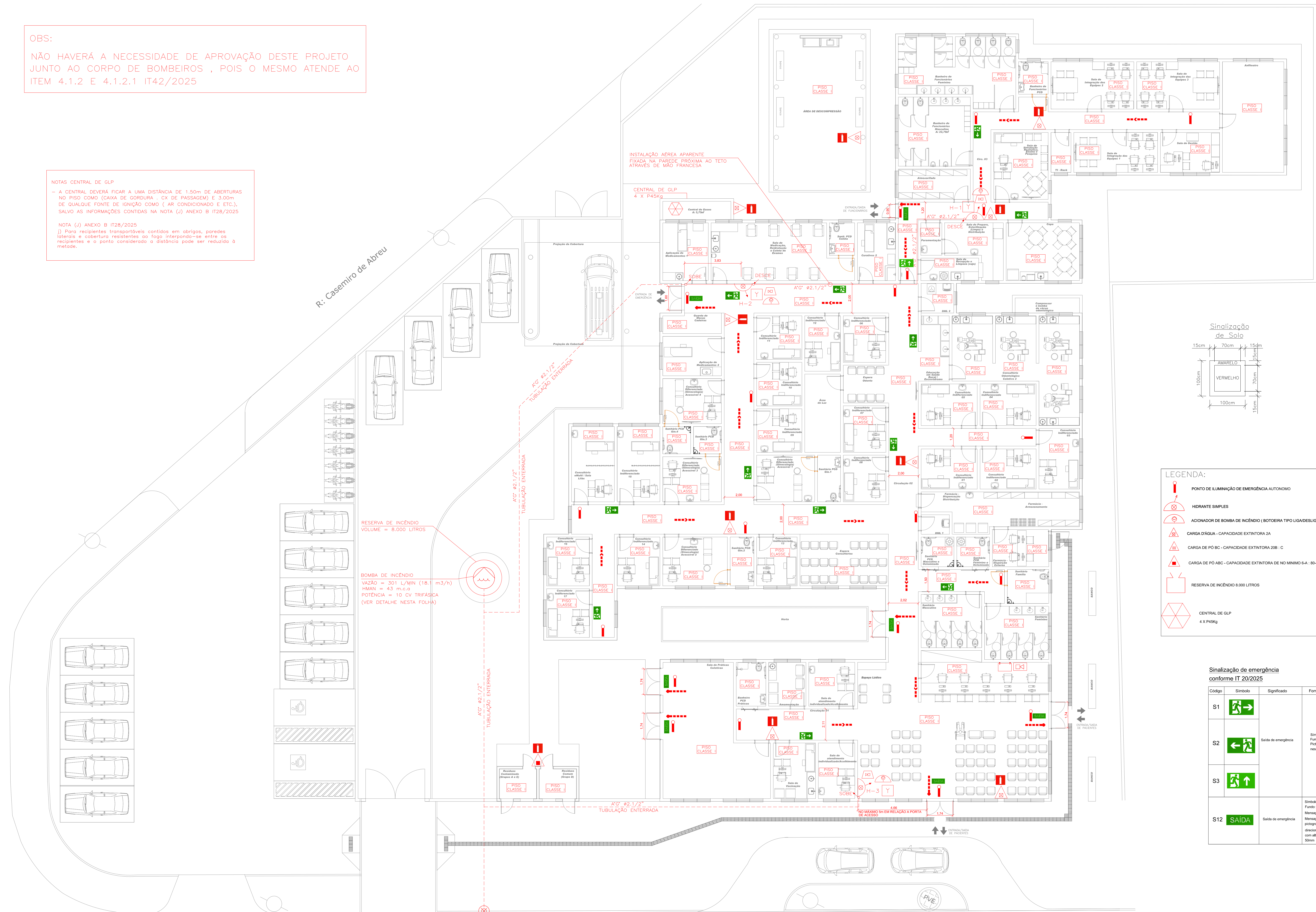
PLANTA BAIXA Escala 1:100
