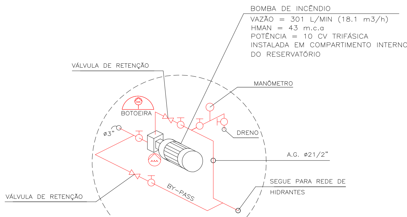
DETALHE A SEM ESCALA
