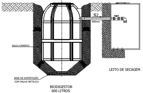
CORTE B-B ESC.: 1:20
