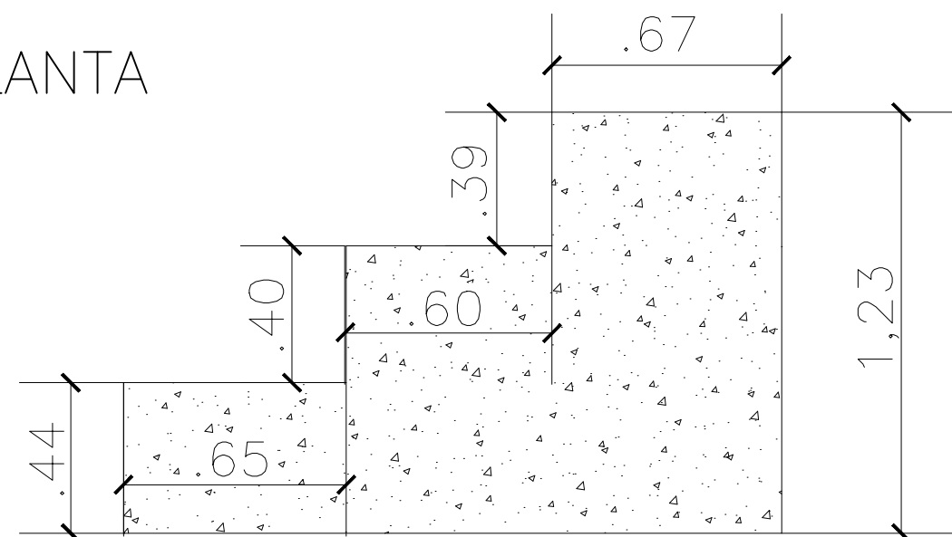
DETALHE ARQUIBANCADA esc. 1/20
