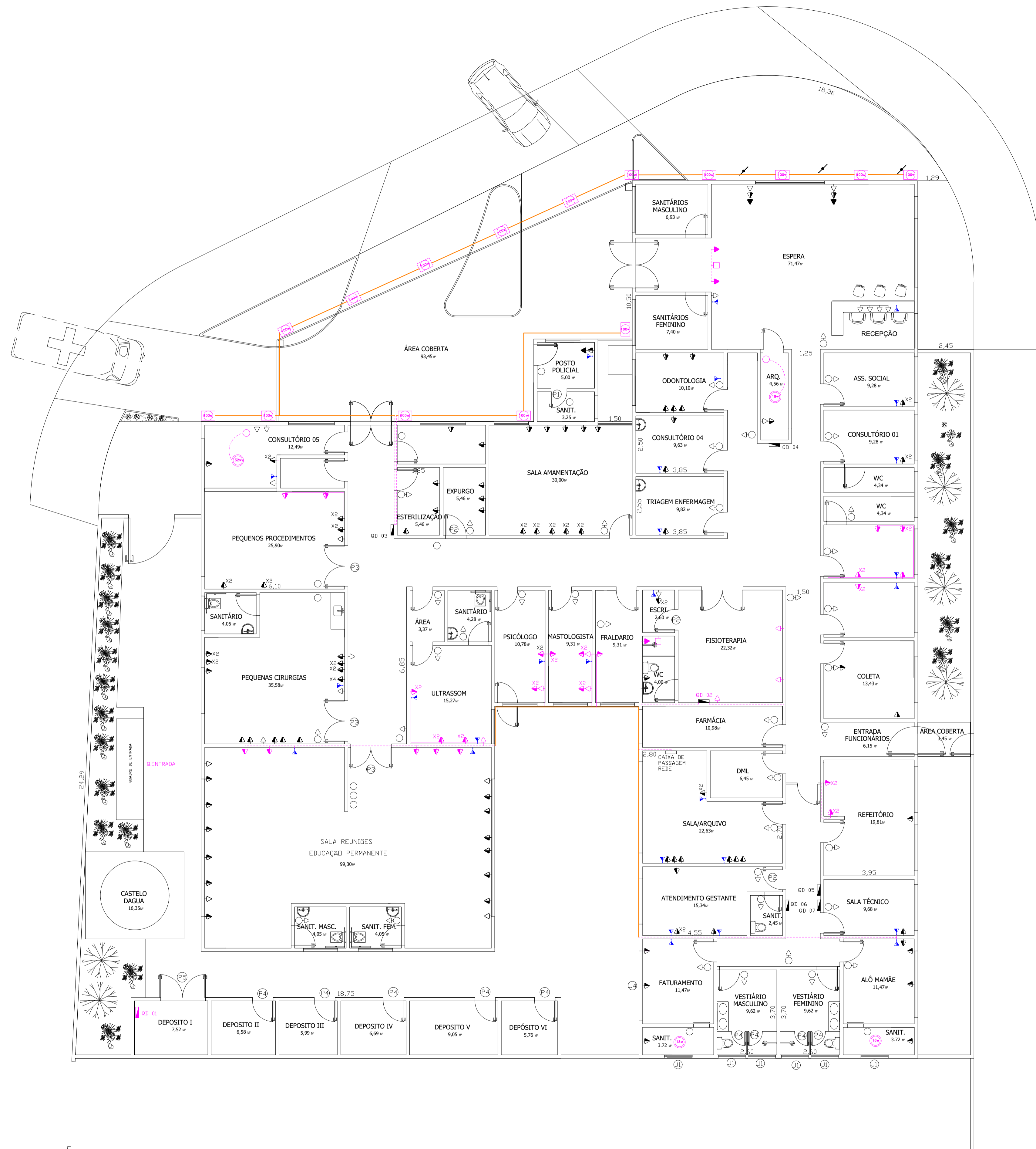
PLANTA PAVIMENTO TÉRREO - READEQUAÇÃO DE PONTOS ELÉTRICOS ESCALA 1:100
