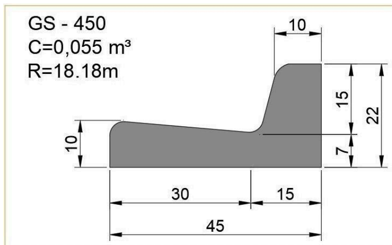
DETALHE - SARJETA E GUIA ESCALA 1:10
