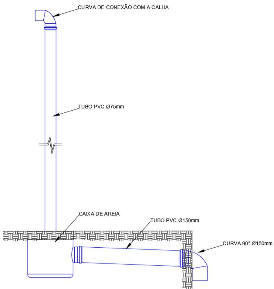
Figura 4 – Croqui da proposta de drenagem
