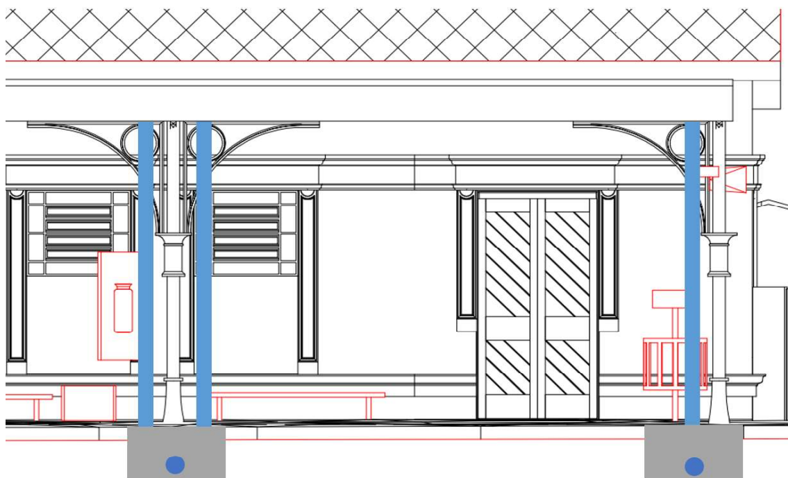
Figura 3 – Croqui de proposta de drenagem
