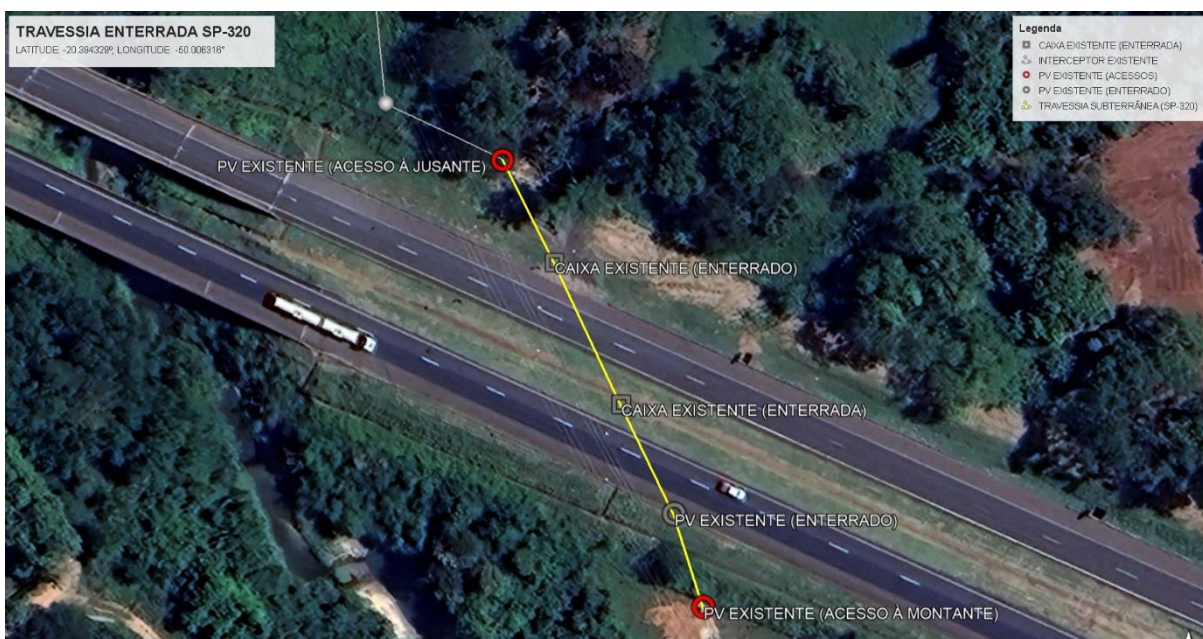
Figura 2: Travessia subterrânea sob a Rodovia Euclides da Cunha (SP-320), km 523.
