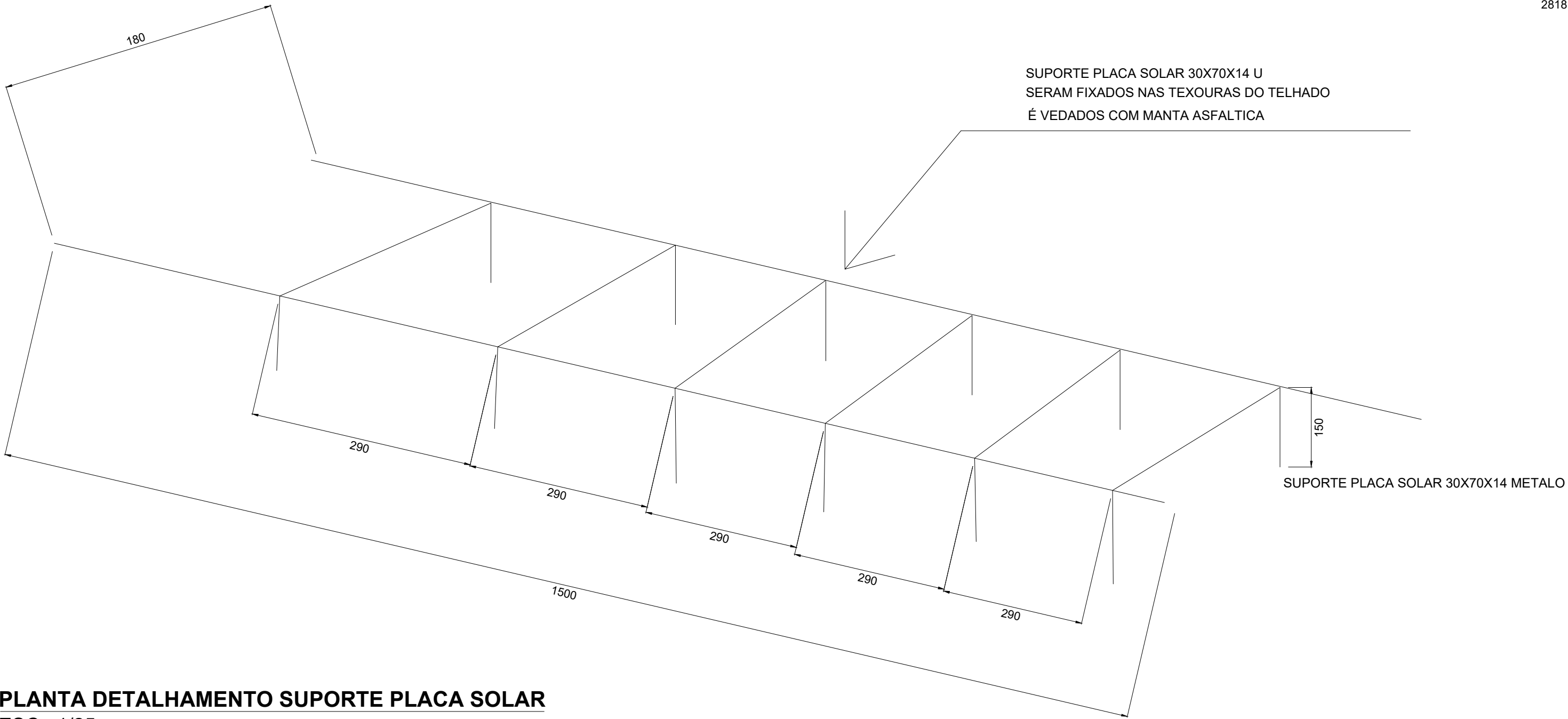
PLANTA DETALHAMENTO SUPORTE PLACA SOLAR ESC.: 1/25
