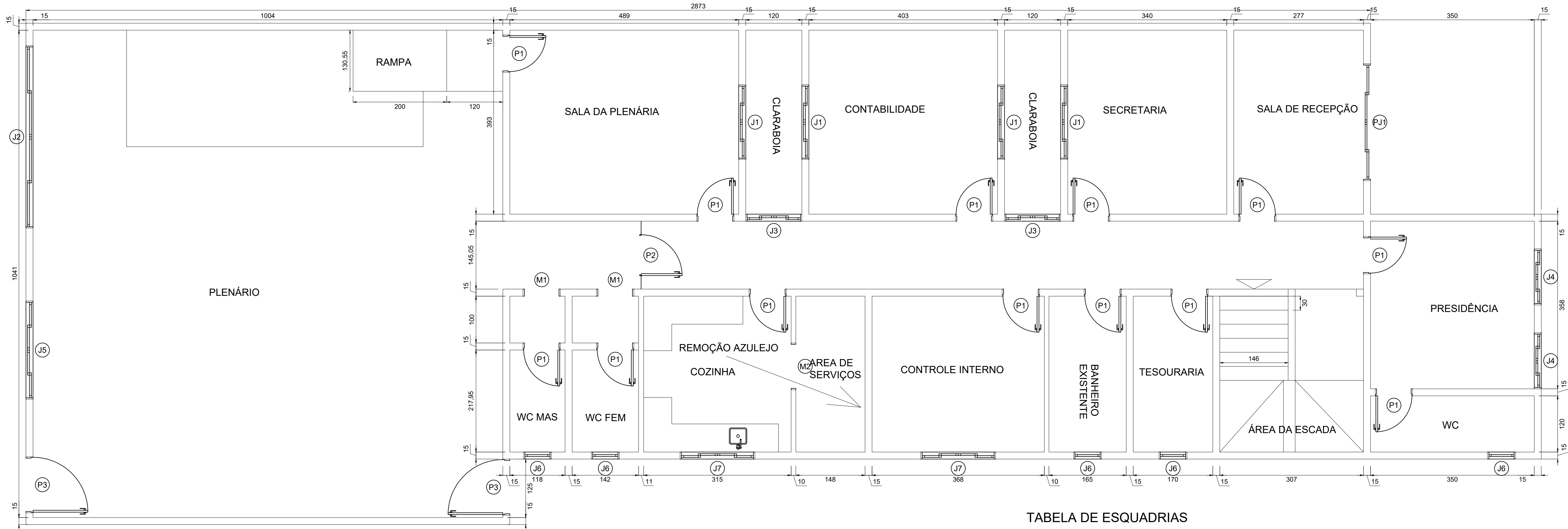
PLANTA BAIXA DO TERREO ESC.: 1/25
