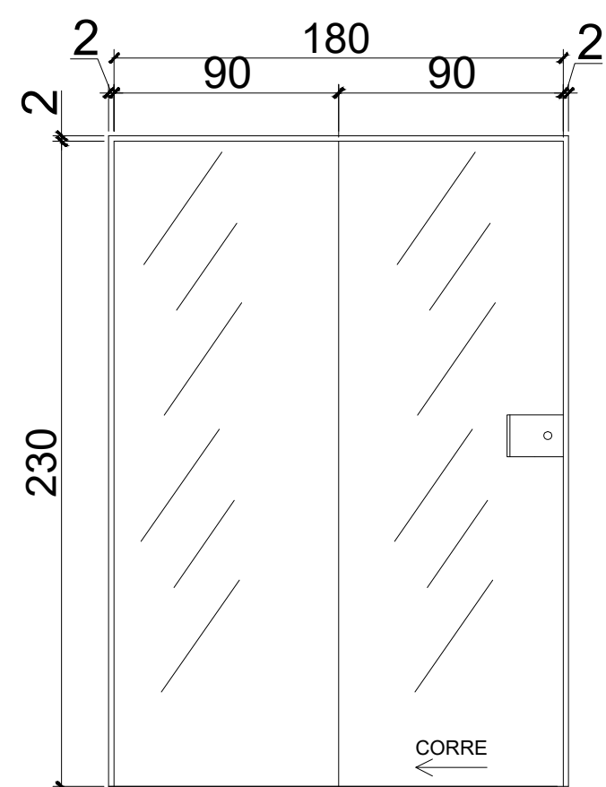
DET. PORTA DE VIDRO ESC.: 1/25
