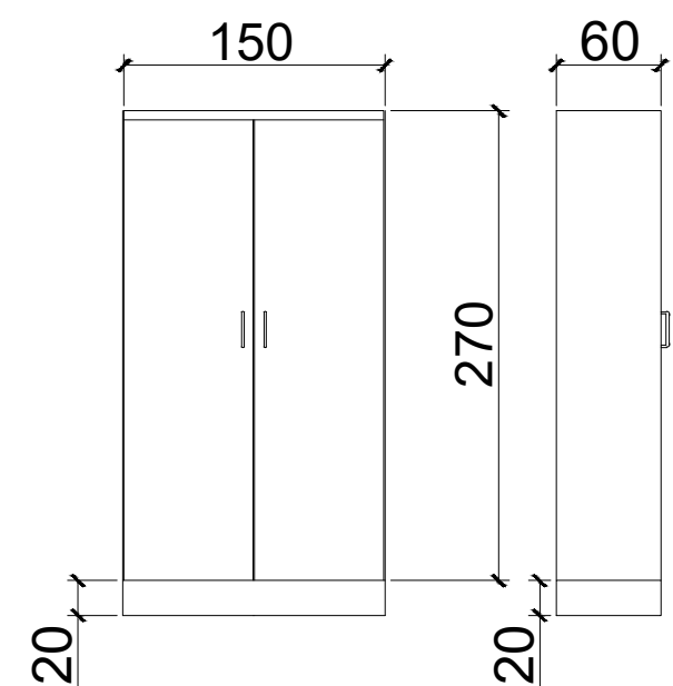
DET.02 ARMARIO DA CENTRAL INTERNET ESC.: 1/25
