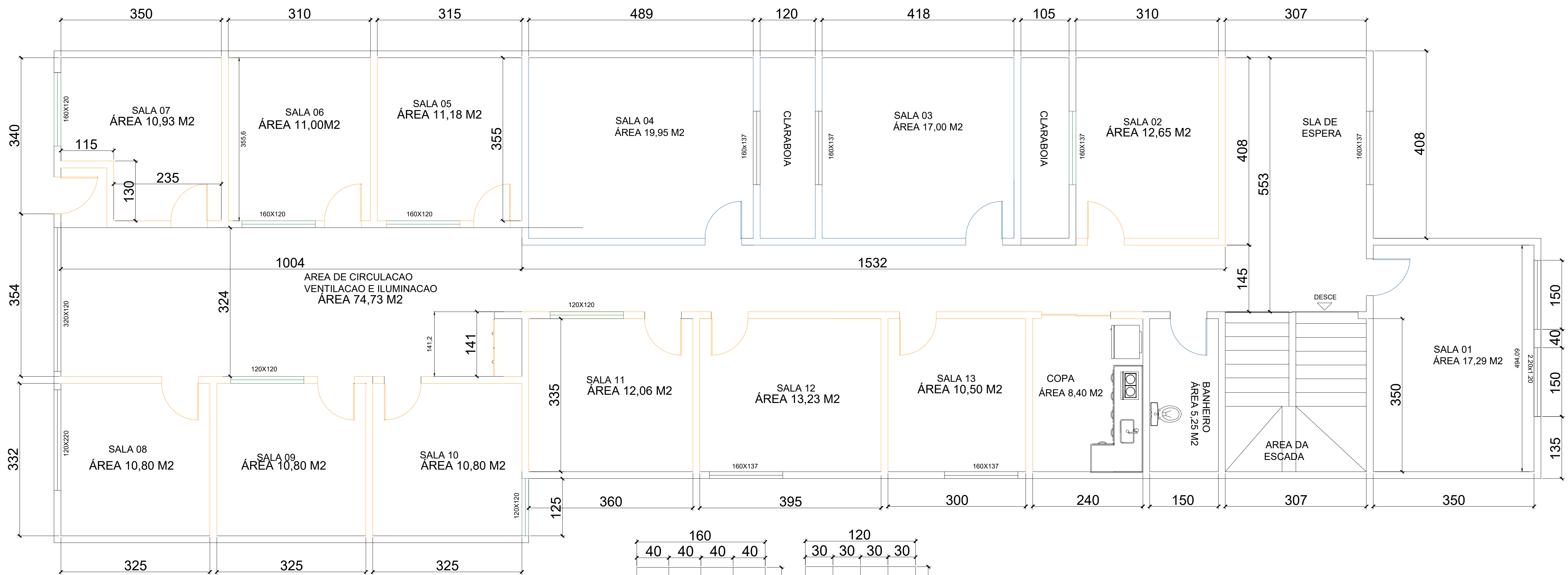
PLANTA BAIXA DO 1 PAV ESC.: 1/25
