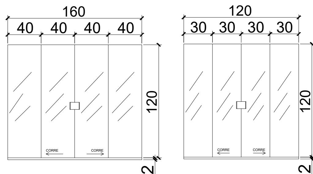
DET. JANELA ESC.: 1/25
