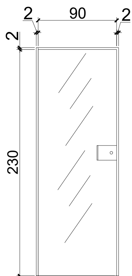
DET. PORTA DE VIDRO ESC.: 1/25
