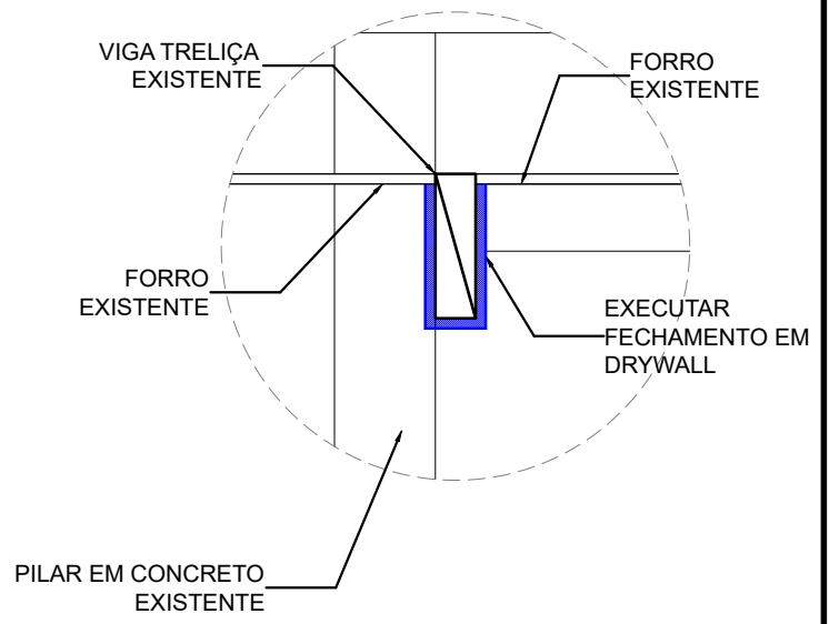
3 DETALHE - VIGA TRELIÇADA ESC 1:25
