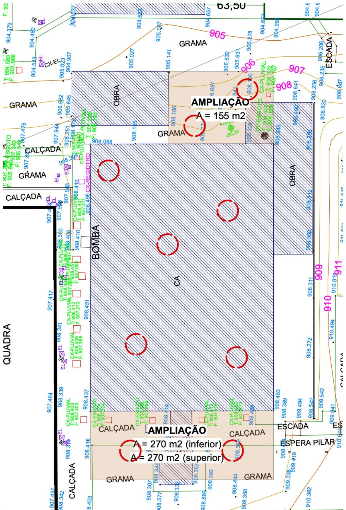
Figura 2 - Locação aproximada dos furos de sondagem nas instalações do edifício do Laboratório Didático de Ginmóricas e Circo do DEDFIS.
